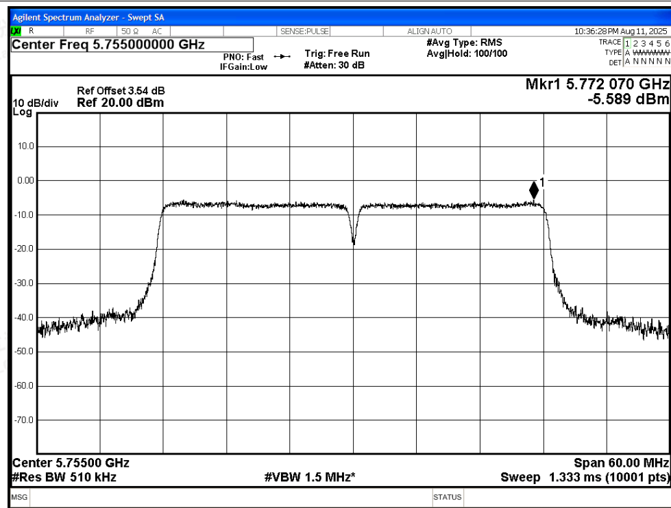
PSD NVNT be40 5755MHz Ant3
