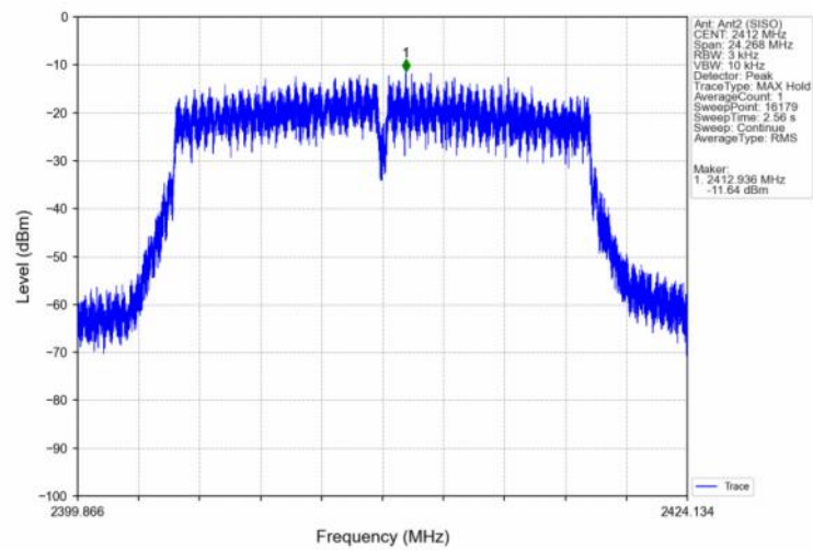
802.11g_LCH_2412MHz_Ant2 (SISO)_NTNV
