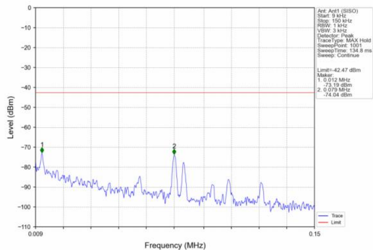
802.11b_LCH_2412MHz_Ant1 (SISO)_NTNV
