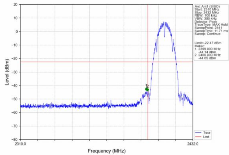
802.11b_LCH_2412MHz_Ant1 (SISO)_NTNV
