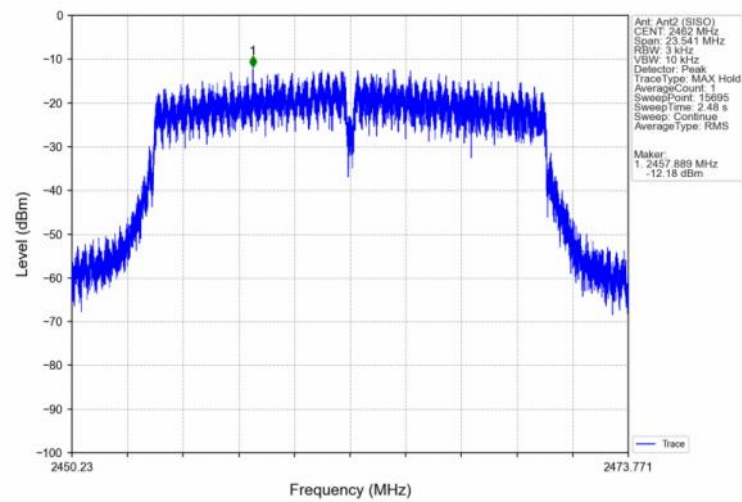
802.11g_HCH_2462MHz_Ant2 (SISO)_NTNV
