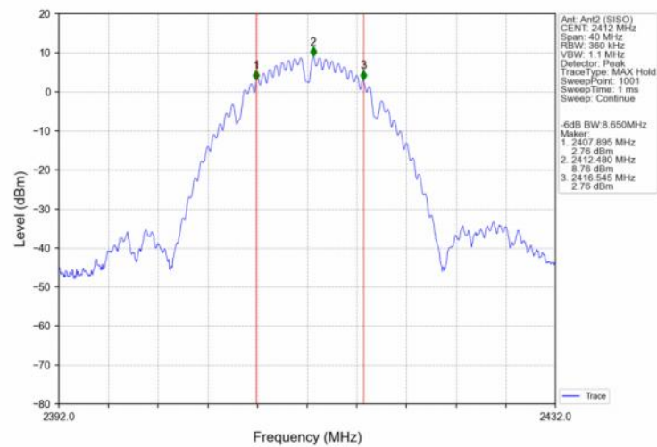
802.11b_LCH_2412MHz_Ant2 (SISO)_NTNV
