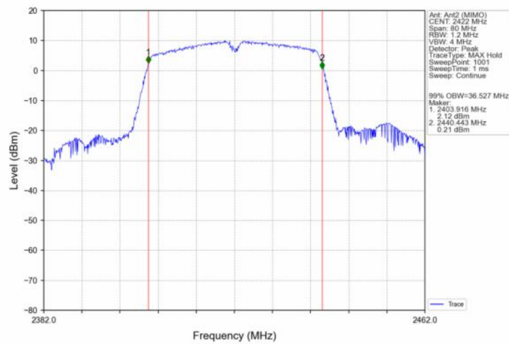
802.11n(HT40)_LCH_2422MHz_Ant2 (MIMO)_NTNV
