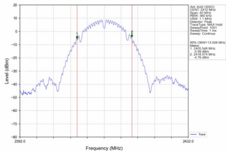
802.11b_LCH_2412MHz_Ant2 (SISO)_NTNV
