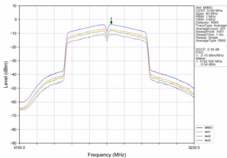
802.11n(HT40) LCH 5190MHz MIMO NTN
