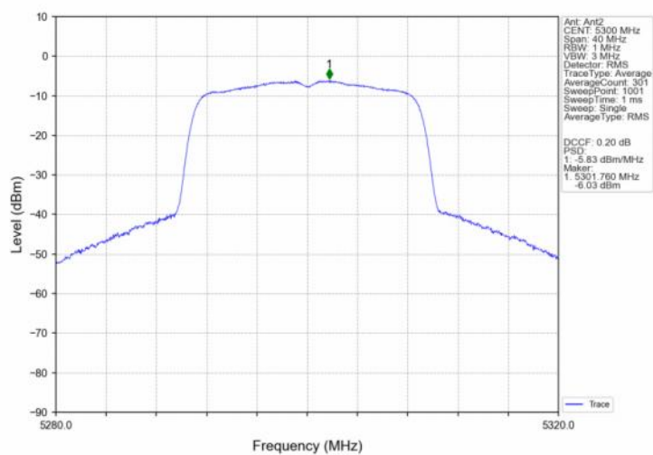
802.11n(HT20) MCH 5300MHz Ant2 NTN
