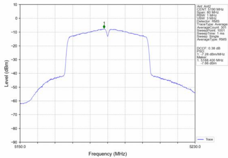
802.11ac(VHT40) LCH 5190MHz Ant2 NTN
