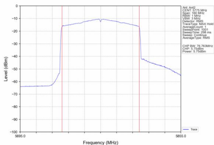
802.11ax(HEW80) MCH 5775MHz SU / Ant2 NTN
