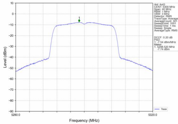
802.11n(HT20) MCH 5300MHz MIMO NTN
