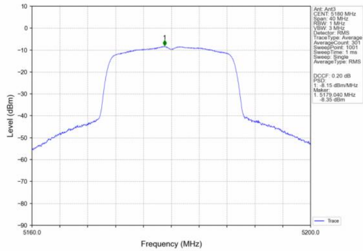
802.11ac(VHT20) LCH 5180MHz MIMO NTN
