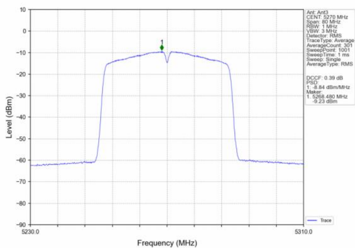
802.11ac(VHT40) LCH 5270MHz MIMO NTN
