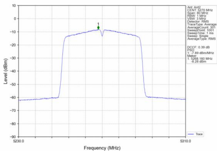
802.11ac(VHT40) LCH 5270MHz Ant2 NTN
