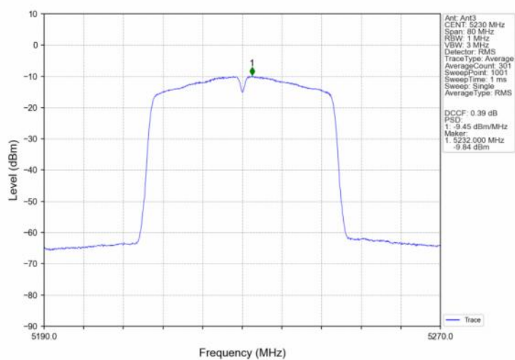
802.11ac(VHT40) HCH 5230MHz MIMO NTN
