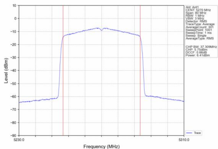
802.11be(EHT40) LCH 5270MHz SU / Ant1 NTN
