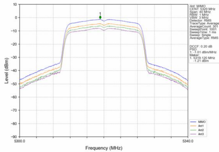
802.11ac(VHT20) HCH 5320MHz MIMO NTN
