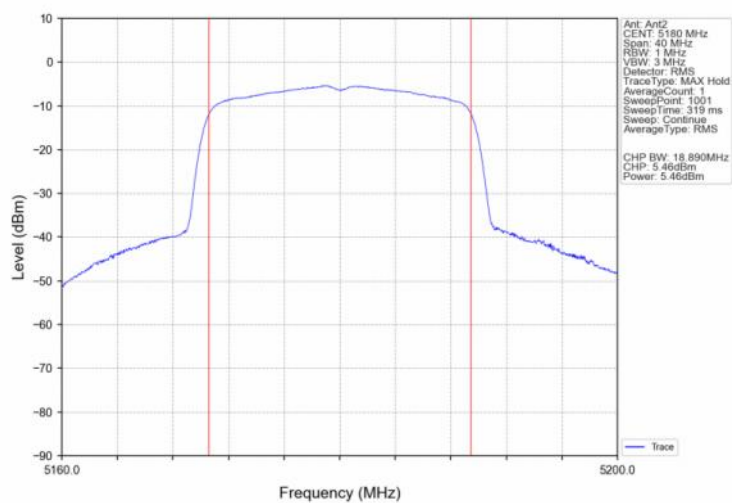
802.11be(EHT20) LCH 5180MHz SU / Ant2 NTV
