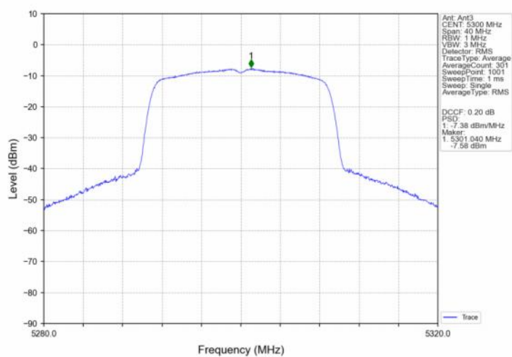
802.11ac(VHT20) MCH 5300MHz MIMO NTN
