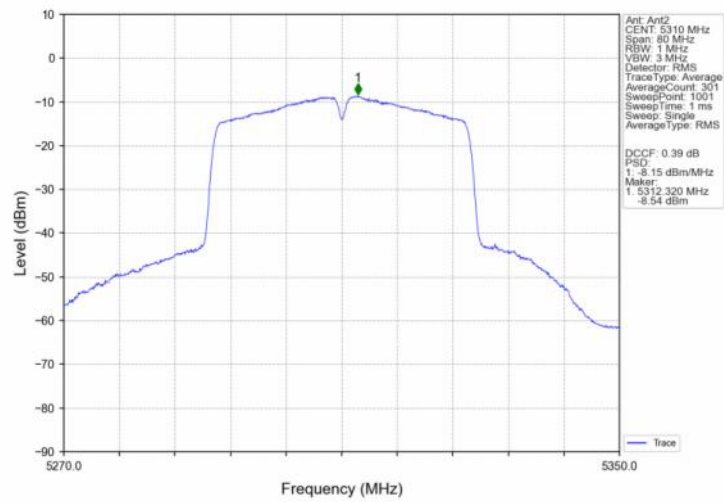
802.11n(HT40) HCH 5310MHz Ant2 NTV
