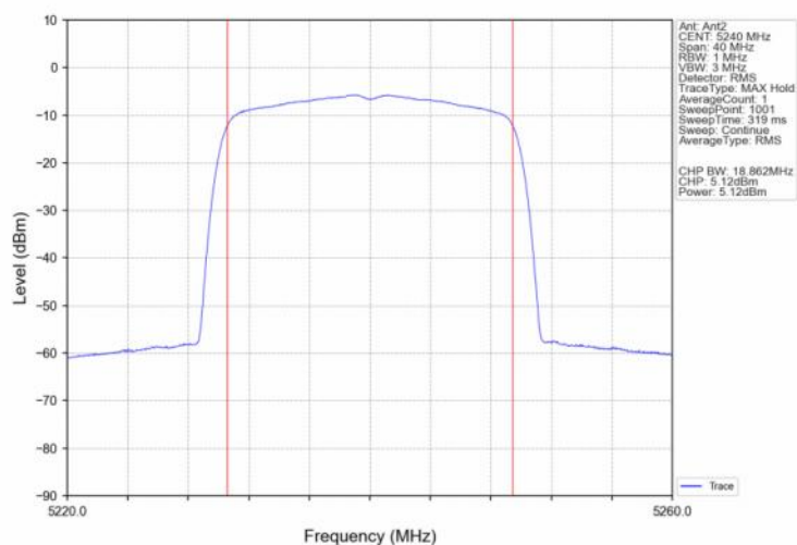
802.11be(EHT20)_HCH_5240MHz_SU_/_Ant2_NTNV
