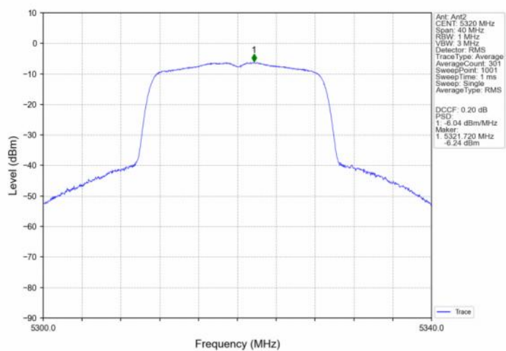
802.11n(HT20) HCH 5320MHz Ant2 NTV
