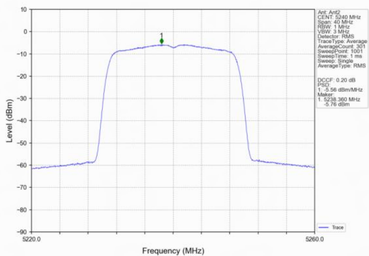
802.11n(HT20) HCH 5240MHz Ant2 NTV
