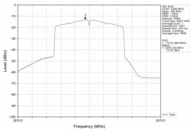
802.11ac(VHT80) MCH 5290MHz MIMO NTN
