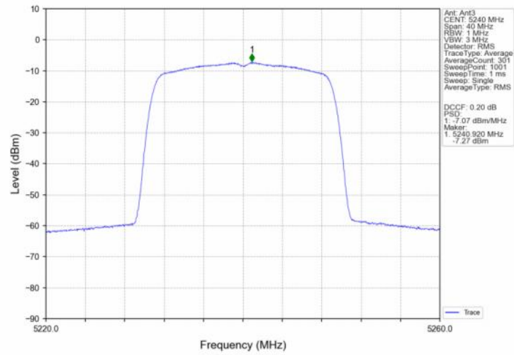
802.11n(HT20) HCH 5240MHz MIMO NTN
