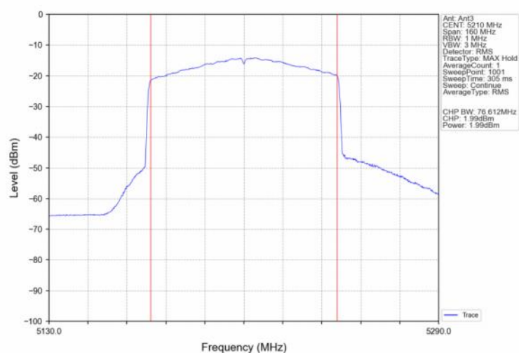
802.11be(EHT80) MCH_5210MHz_SU / Ant3 NTN
