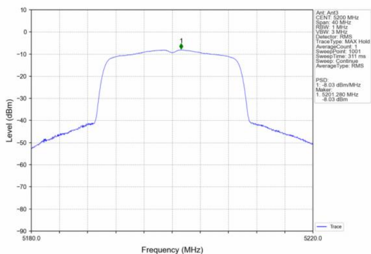
802.11ax(HEW20) MCH 5200MHz SU / MIMO NTN
