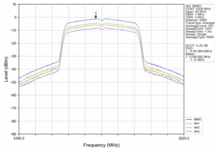
802.11ac(VHT20) MCH 5200MHz MIMO NTN
