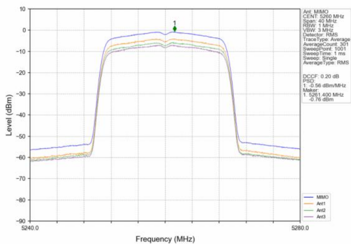
802.11ac(VHT20) LCH 5260MHz MIMO NTN
