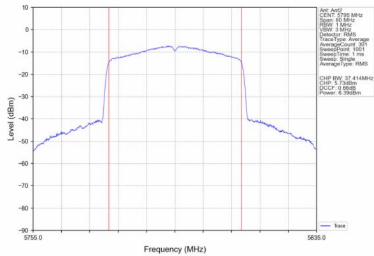
802.11be(EHT40) HCH_5795MHz_SU / Ant2_NTNV
