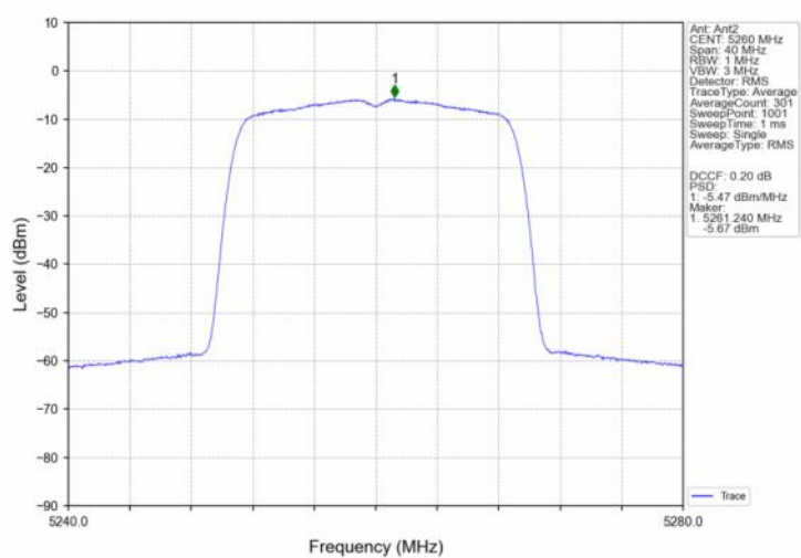
802.11ac(VHT20) LCH 5260MHz Ant2 NTN
