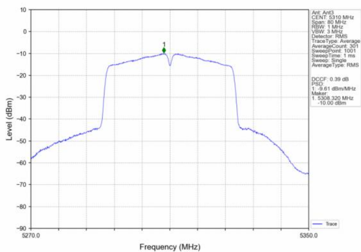
802.11ac(VHT40) HCH 5310MHz MIMO NTN
