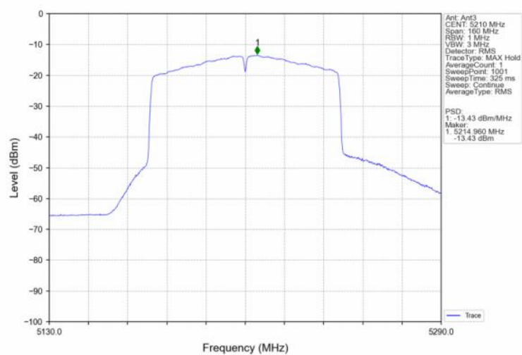
802.11ac(VHT80) MCH 5210MHz MIMO NTN
