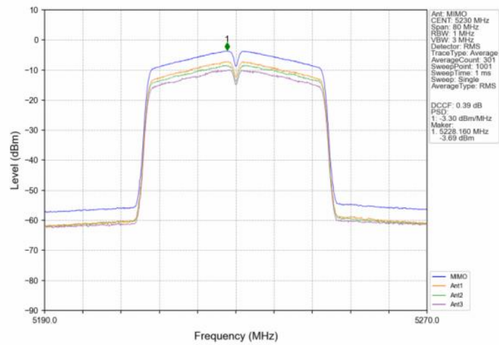
802.11n(HT40) HCH 5230MHz MIMO NTN
