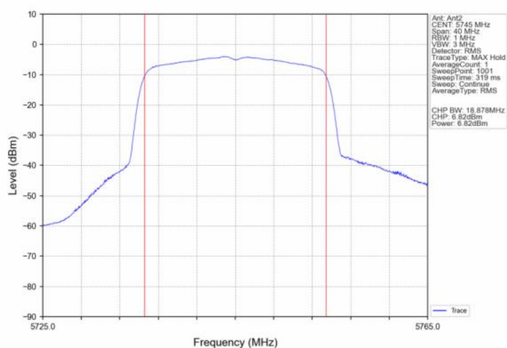
802.11be(EHT20) LCH 5745MHz SU / Ant2 NTNV
