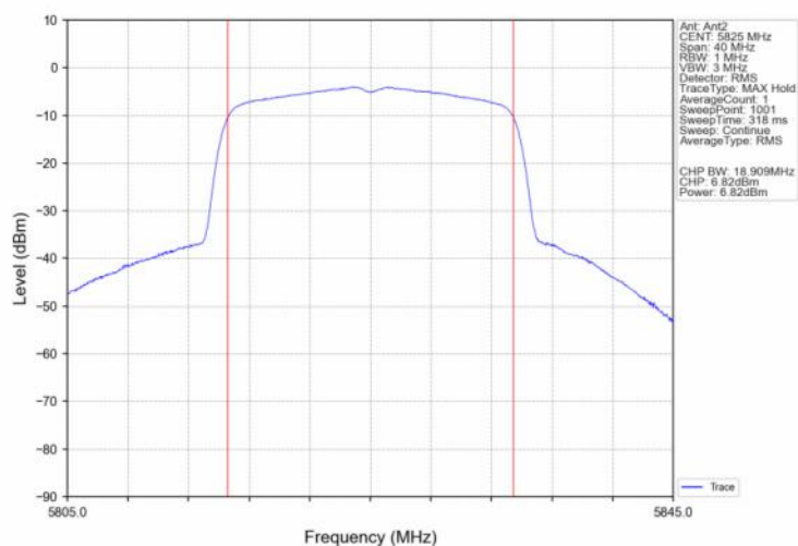
802.11be(EHT20)_HCH_5825MHz_SU / Ant2_NTNV
