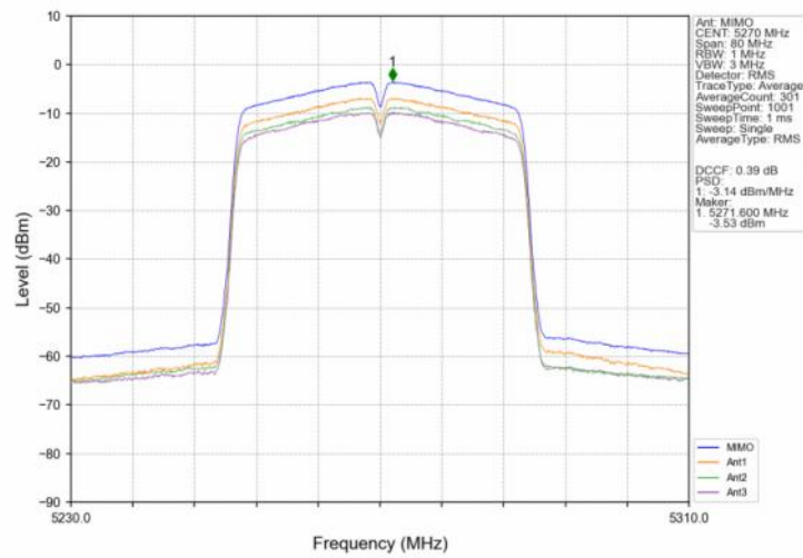
802.11n(HT40) LCH 5270MHz MIMO NTN
