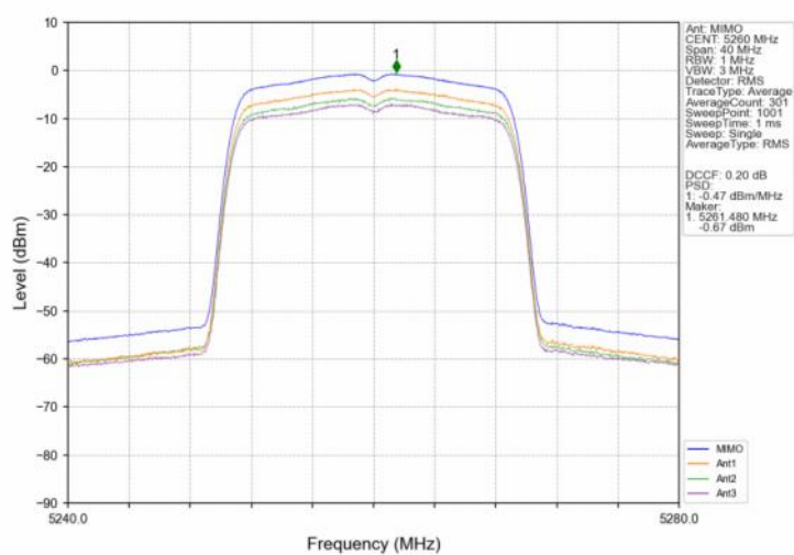
802.11n(HT20) LCH 5260MHz MIMO NTN
