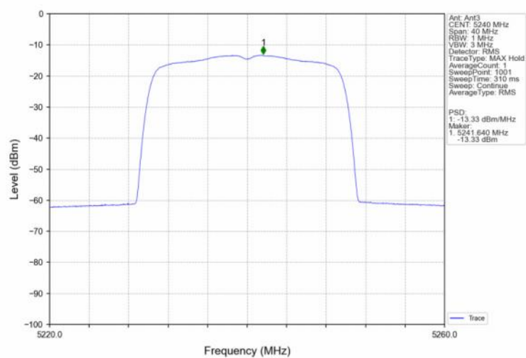
802.11ax(HEW20) HCH 5240MHz SU / MIMO NTN
