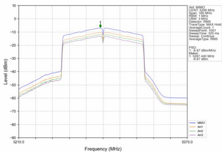
802.11ac(VHT80) MCH 5290MHz MIMO NTN
