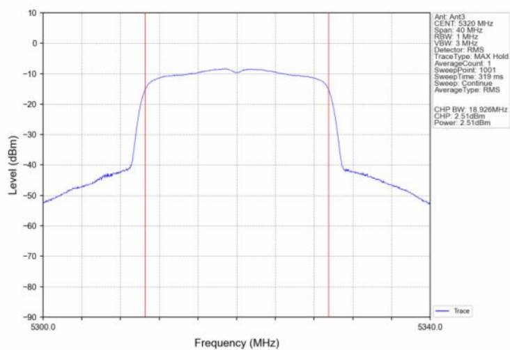
802.11be(EHT20)_HCH_5320MHz_SU / Ant3_NTNV
