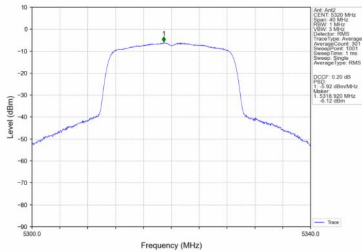
802.11ac(VHT20) HCH 5320MHz Ant2 NTN
