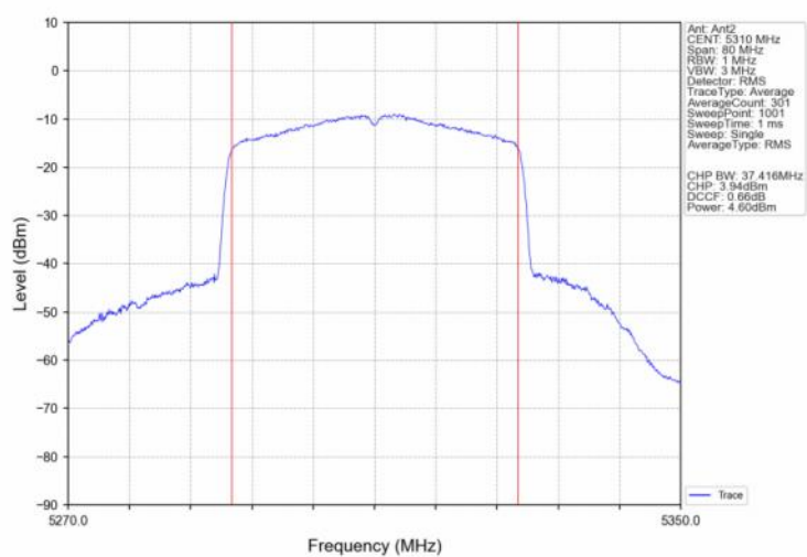
802.11be(EHT40) HCH_5310MHz_SU / Ant2_NTNV
