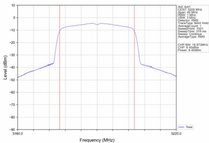
802.11be(EHT20) MCH 5200MHz SU / Ant1 NTN
