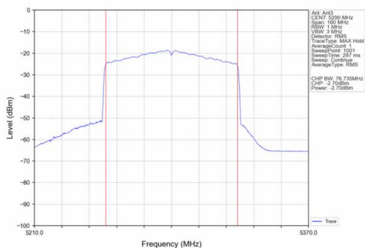
802.11ax(HEW80) MCH 5290MHz SU / Ant3 NTN
