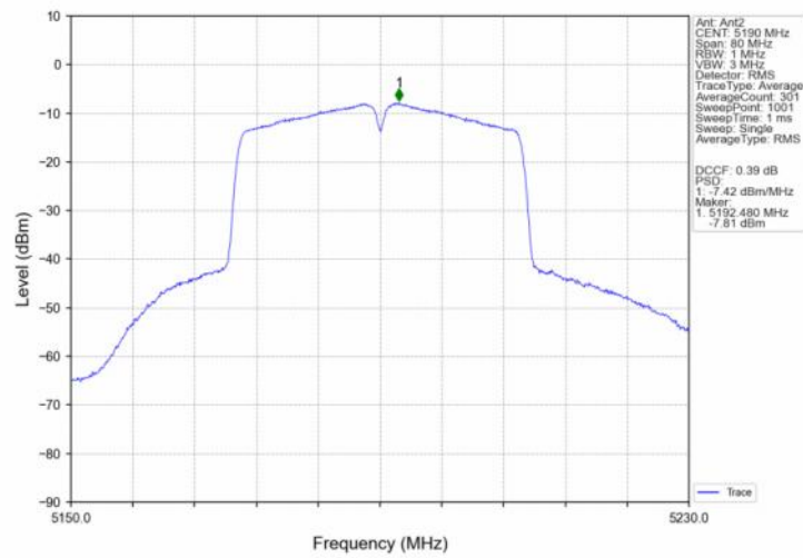
802.11n(HT40) LCH 5190MHz Ant2 NTN
