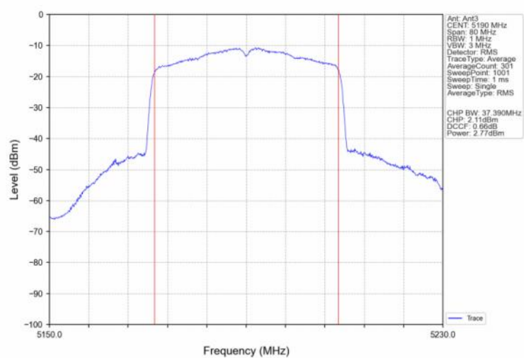
802.11be(EHT40) LCH 5190MHz SU / Ant3 NTNV
