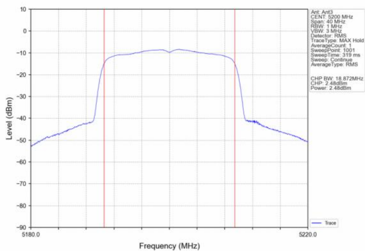
802.11be(EHT20) MCH_5200MHz_SU / Ant3 NTN
