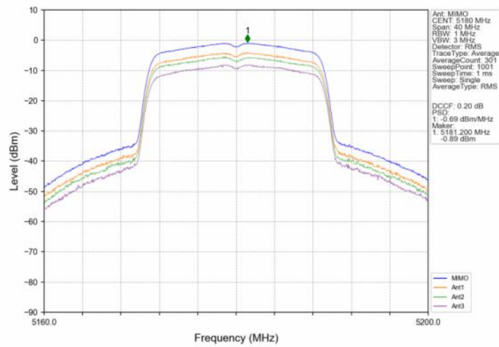
802.11n(HT20) LCH 5180MHz MIMO NTN
