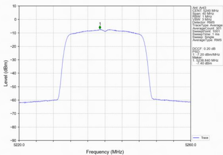
802.11ac(VHT20) HCH 5240MHz MIMO NTN
