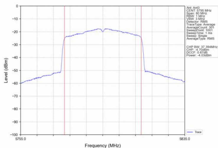
802.11ax(HEW40) HCH 5795MHz SU / Ant3 NTN
