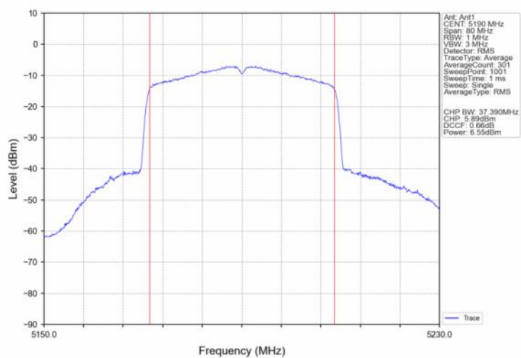
802.11be(EHT40) LCH 5190MHz SU / Ant1 NTN
