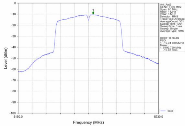
802.11ac(VHT40) LCH 5190MHz MIMO NTN
