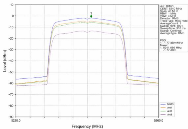
802.11ax(HEW20) HCH 5240MHz SU / MIMO NTN
