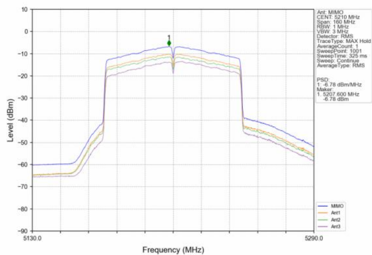
802.11ac(VHT80) MCH 5210MHz MIMO NTN
