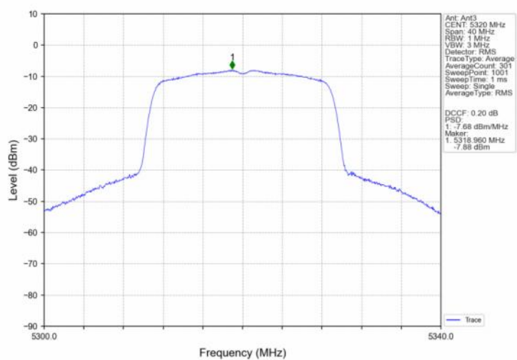
802.11n(HT20) HCH 5320MHz MIMO NTN
