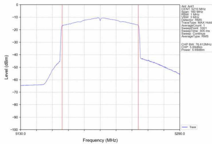
802.11be(EHT80) MCH 5210MHz SU / Ant1 NTNv
