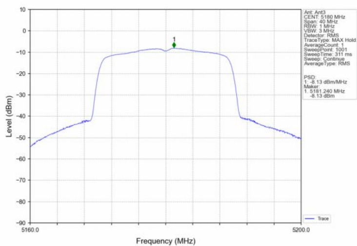
802.11ax(HEW20) LCH 5180MHz SU / MIMO NTN
