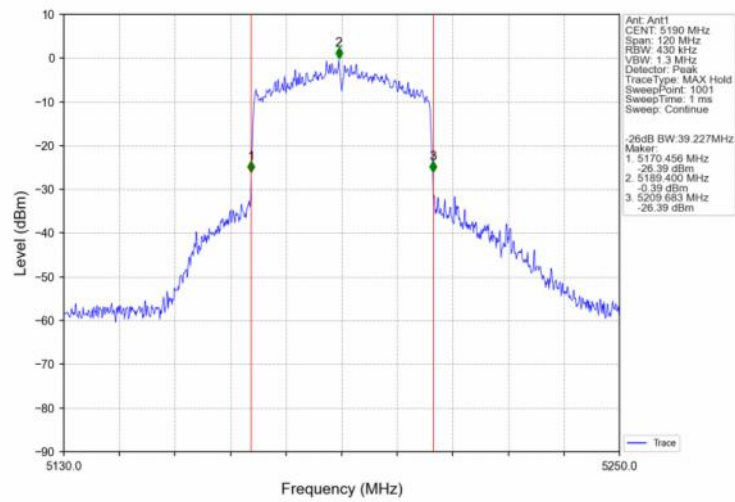
802.11ax(HEW40) LCH 5190MHz SU / Ant1 NTN
