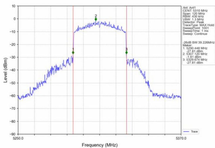
802.11be(EHT40) HCH 5310MHz SU / Ant1 NTN
