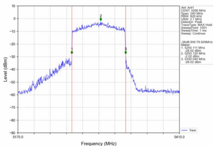
802.11be(EHT80) MCH_5290MHz_SU / Ant1 NTNv
