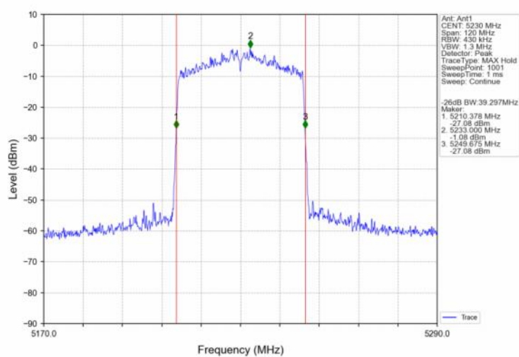
802.11be(EHT40) HCH 5230MHz SU / Ant1 NTN
