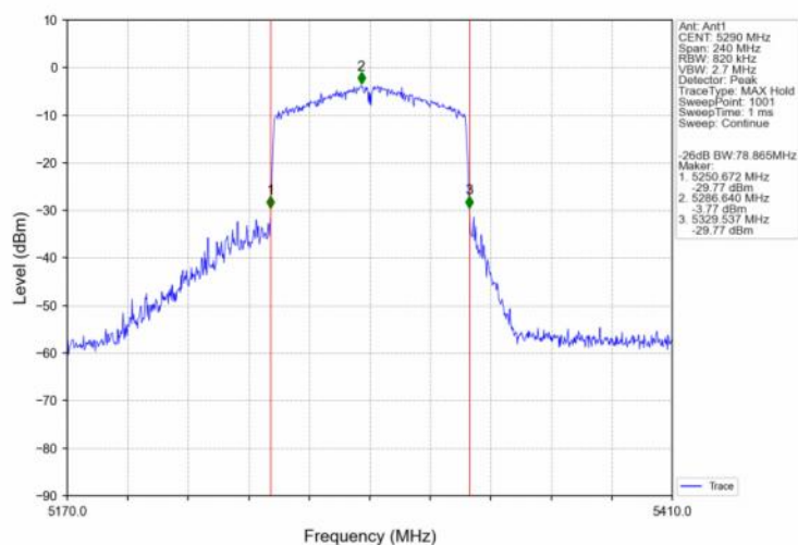
802.11ac(VHT80) MCH 5290MHz Ant1 NTN
