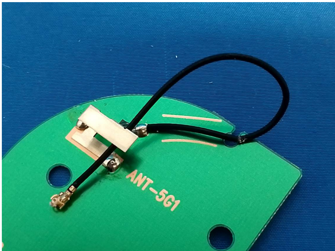
5GWifi Antenna(Chain 0)
