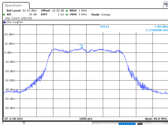
802.11ac20_5280MHz_Chain 1
