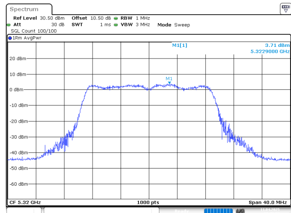
802.11ac20_5320MHz_Chain 1
