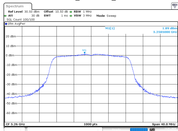
802.11n20_5260MHz_Chain 0
