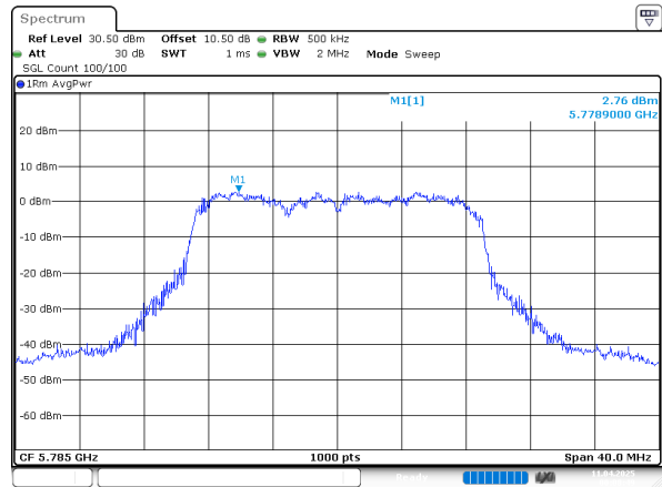
802.11ac20_5785MHz_Chain 0
