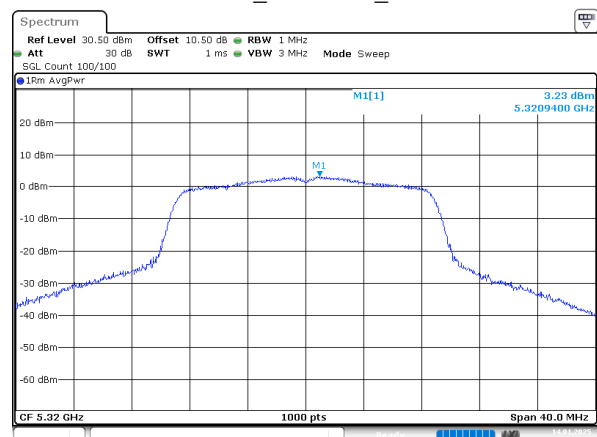
802.11n20_5320MHz_Chain 0
