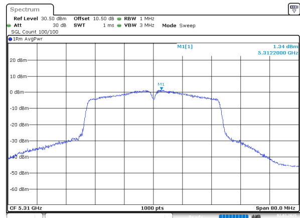
802.11n40_5310MHz_Chain 2
