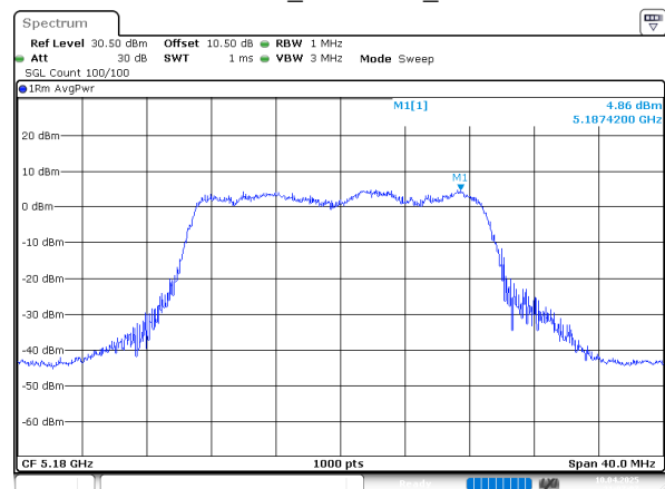
802.11ac20_5180MHz_Chain 1
