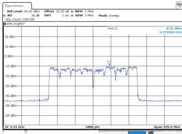
802.11ac160_5250MHz_Chain 2
