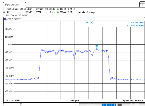
802.11ac80_5210MHz_Chain 0
