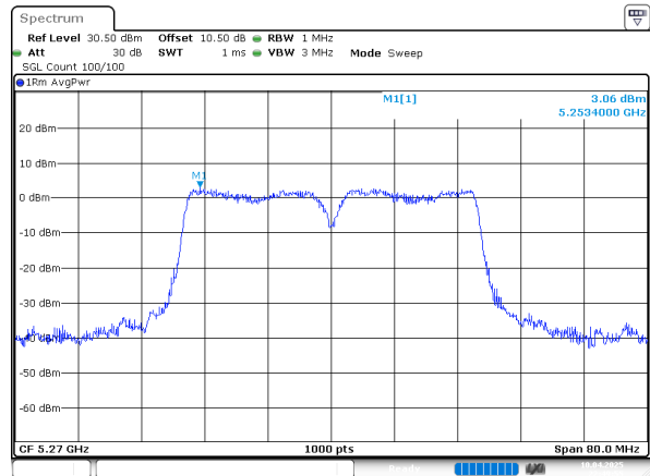
802.11ac40_5270MHz_Chain 2
