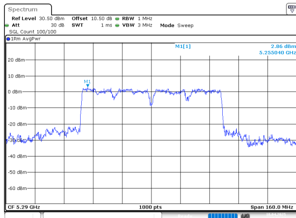
802.11ac80_5290MHz_Chain 1
