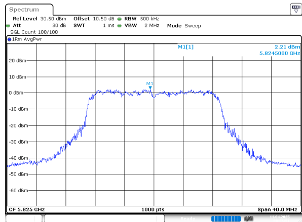
802.11ac20_5825MHz_Chain 1
