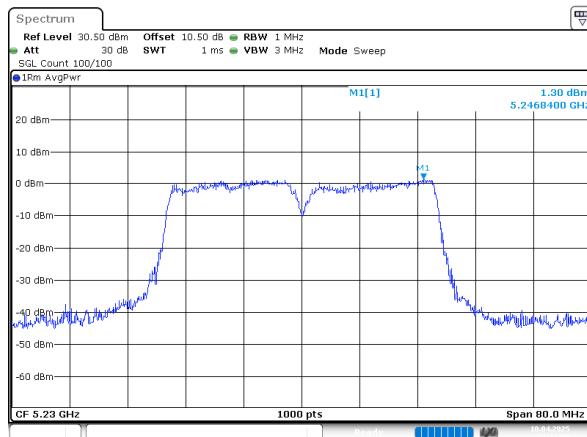
802.11ac40_5230MHz_Chain 2
