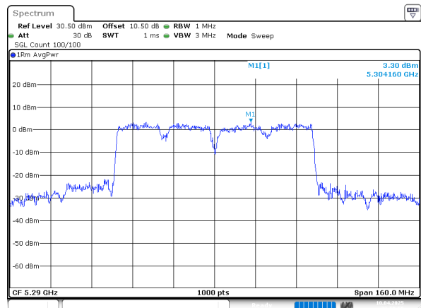
802.11ac80_5290MHz_Chain 2
