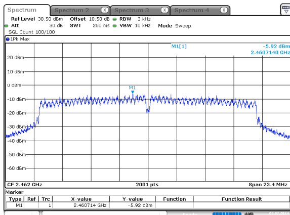
n20_2462MHz_Chain 0
