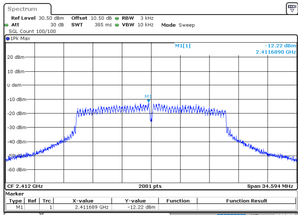
802.11n20_2412MHz
