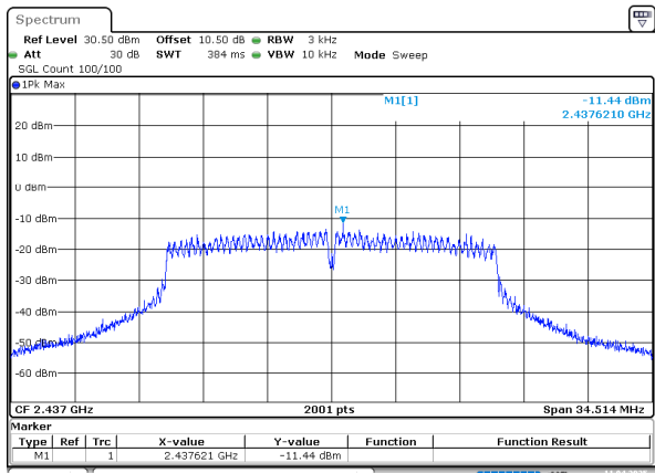
802.11n20_2437MHz
