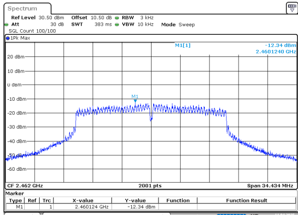
802.11n20_2462MHz
