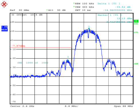
802.11b_2412MHz_Chain 1
