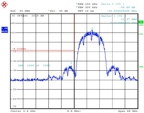
802.11b_2412MHz_Chain 0
