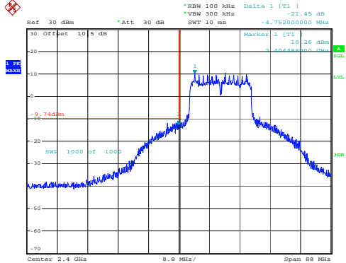
802.11n20_2412MHz_Chain 0
