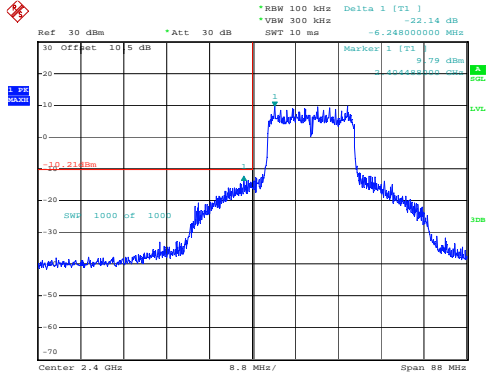
802.11n20_2412MHz_Chain 1
