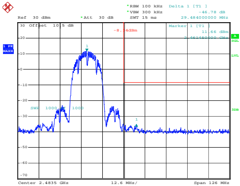
802.11b_2462MHz_Chain 1
