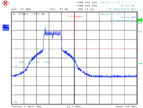
802.11n20_2462MHz_Chain 0
