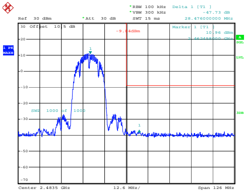
802.11b_2462MHz_Chain 0
