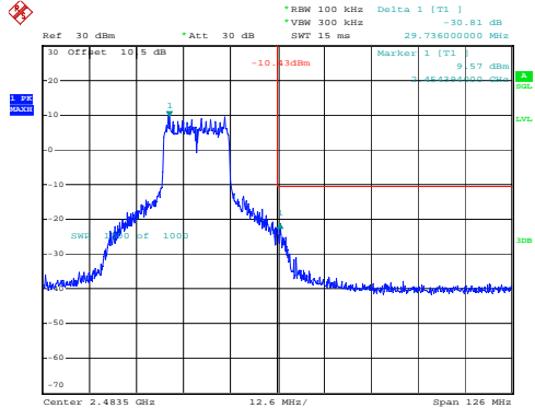
802.11n20_2462MHz_Chain 1
