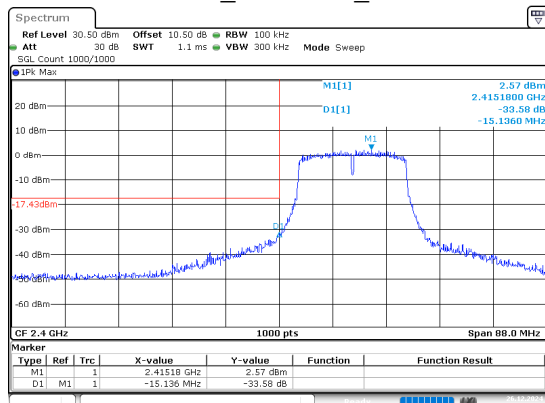
802.11n20_2412MHz_Chain 1
