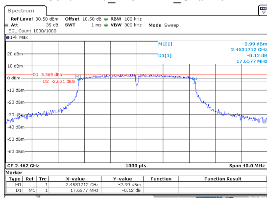
802.11n20_2462MHz_Chain 0
