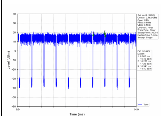
802.11n (HT20)
