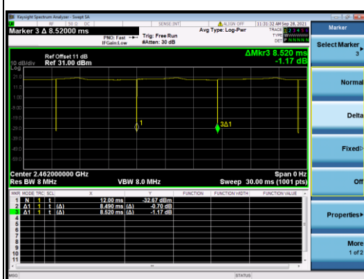
802.11n (HT20)
