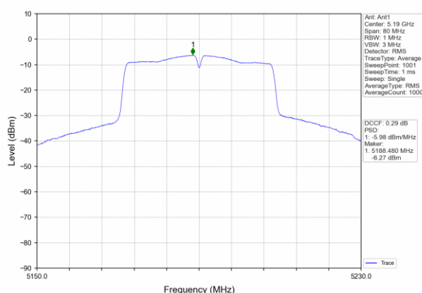
802.11ac (40MHz)
