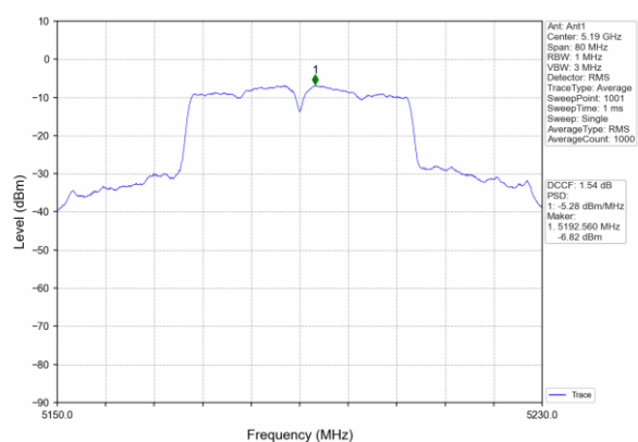
802.11ac (40MHz)
