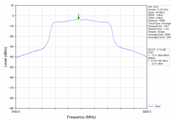
802.11ac (20MHz)
