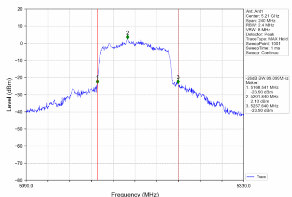
802.11ac (80MHz)
