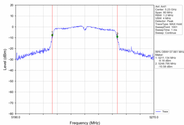
802.11ac (40MHz)
