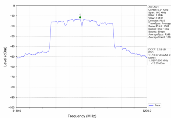
802.11ac (80MHz)
