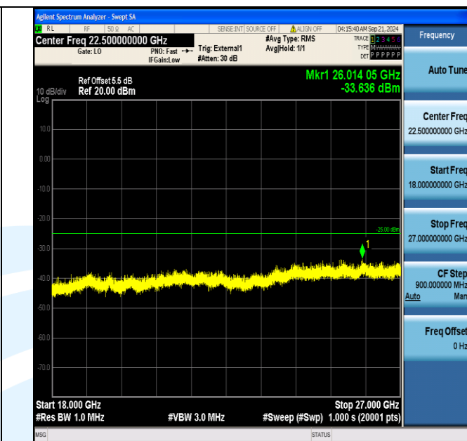
Band41_10MHz_QPSK_40690_50RB#0_18000~27000_18000~27000
