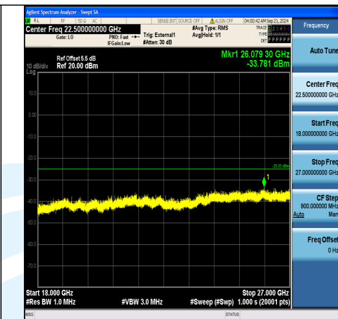
Band41_10MHz_16QAM_40290_1RB#0_18000~27000_18000~27000
