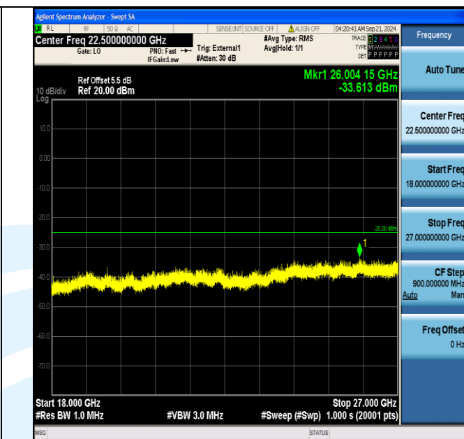
Band41_10MHz_16QAM_41190_1RB#0_18000~27000_18000~27000
