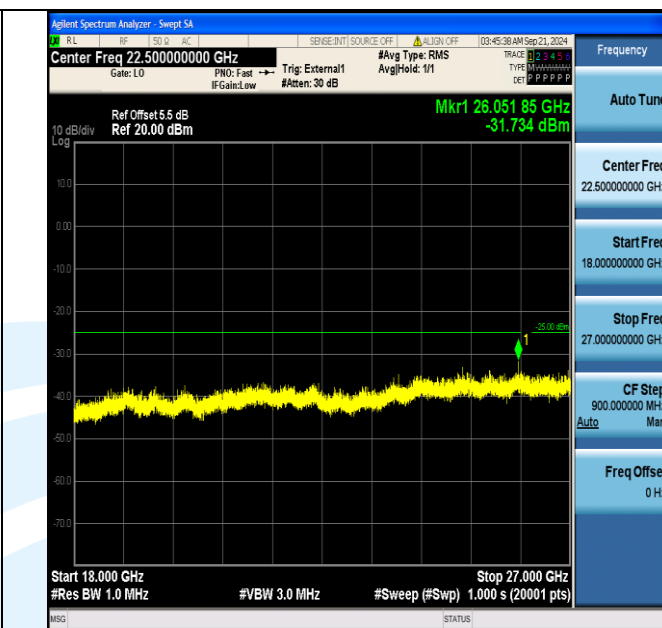
Band41_5MHz_QPSK_40690_25RB#0_18000~27000_18000~27000
