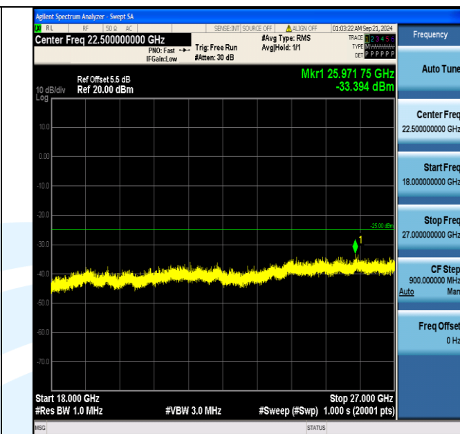
Band7_15MHz_16QAM_21100_1RB#0_18000~27000_18000~27000
