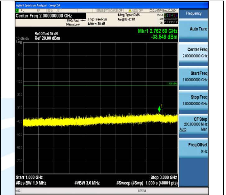
Band5 3MHz QPSK 20635 15RB#0 1000~3000 1000~3000
