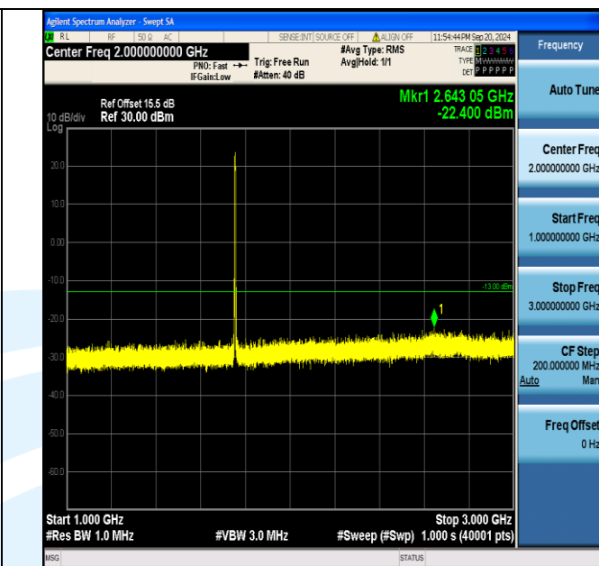
Band4 3MHz QPSK 20385 15RB#0 1000~3000 1000~3000
