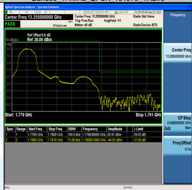
Band66 1.4MHz QPSK 132665 1RB#0
