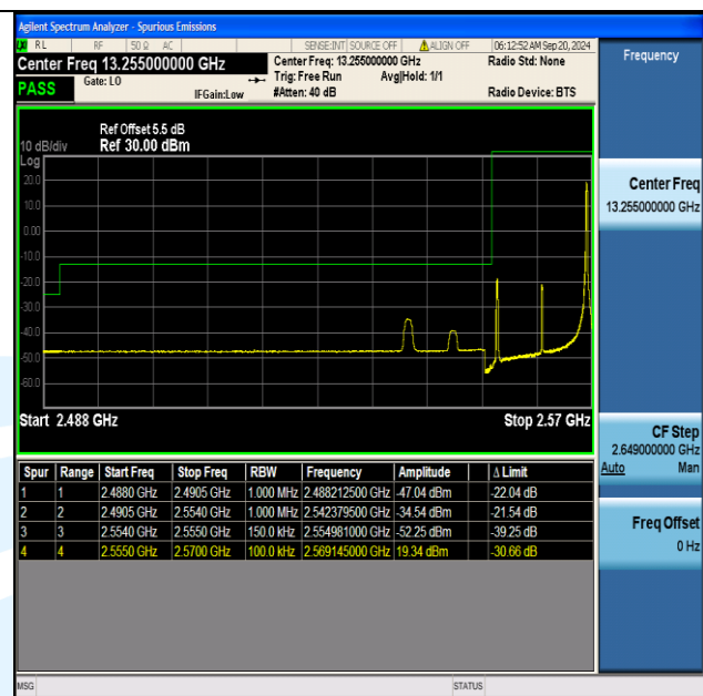
Band41 15MHz QPSK 40315 1RB#74
