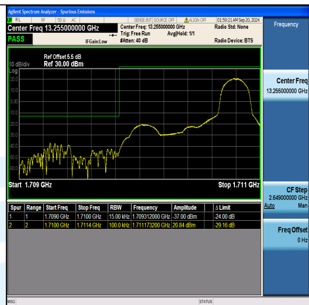
Band66 1.4MHz QPSK 131979 1RB#5
