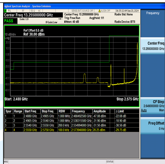
Band41 20MHz QPSK 40340 1RB#99
