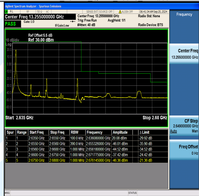
Band41 20MHz QPSK 41140 1RB#0
