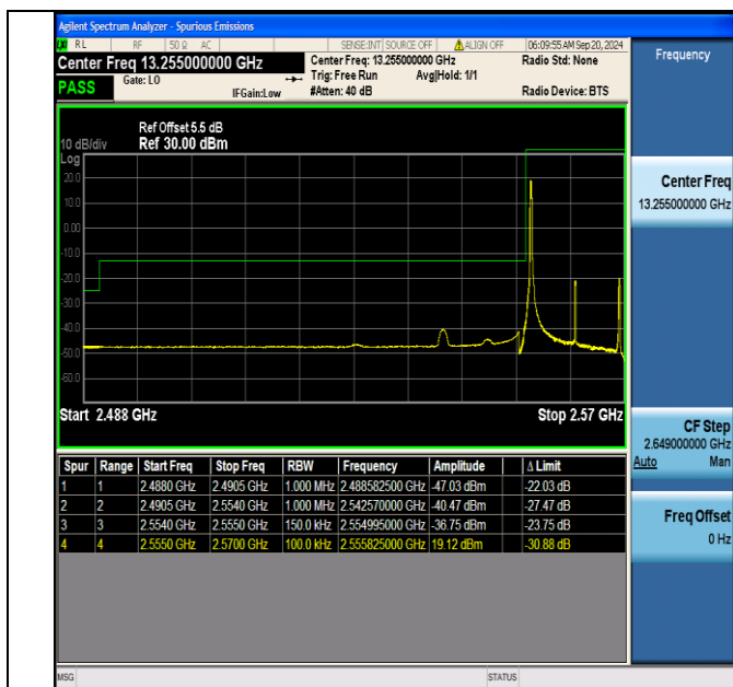
Band41 15MHz QPSK 40315 1RB#0
