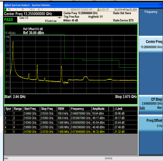
Band41 15MHz QPSK 41165 1RB#0
