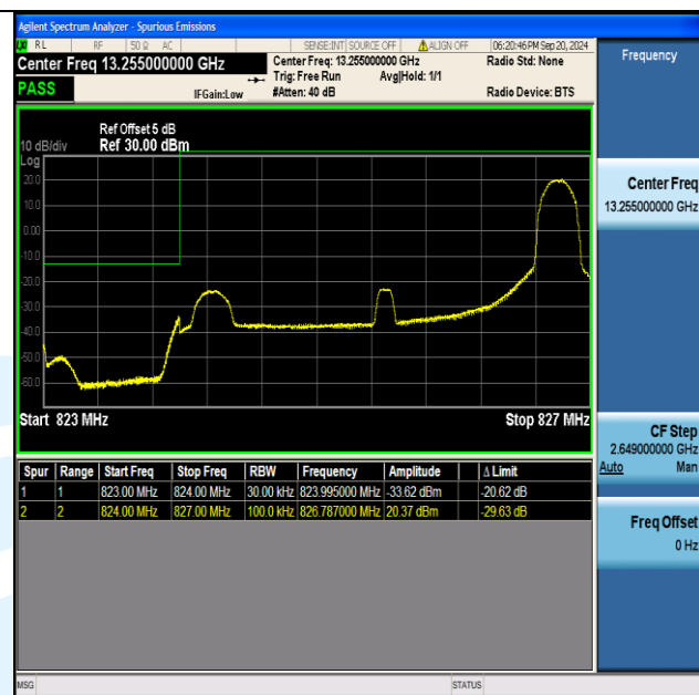
Band5 3MHz QPSK 20415 1RB#14
