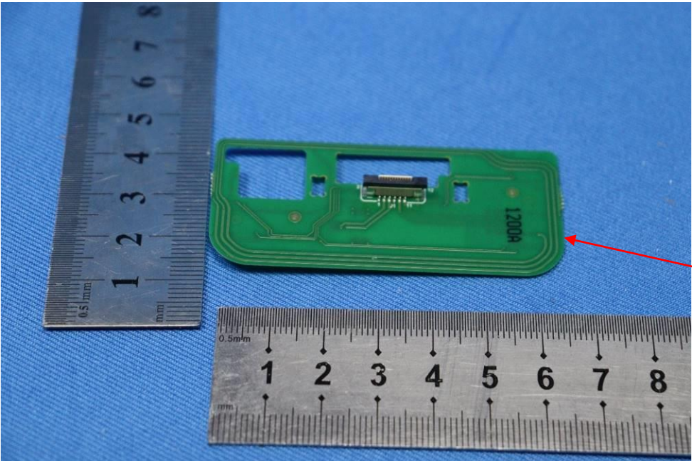
NFC Antenna
