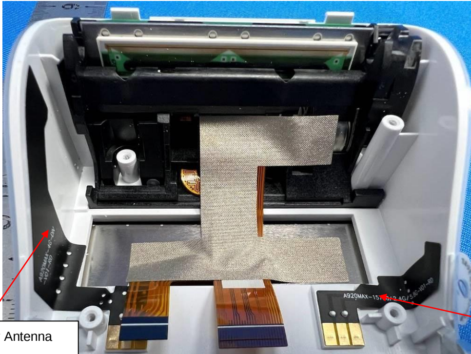
BT/WiFi/GPS Antenna
