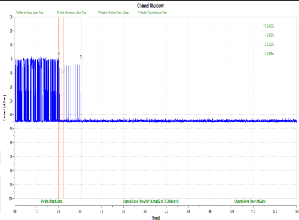
11AC80SISO-5290-Type0-PASS
