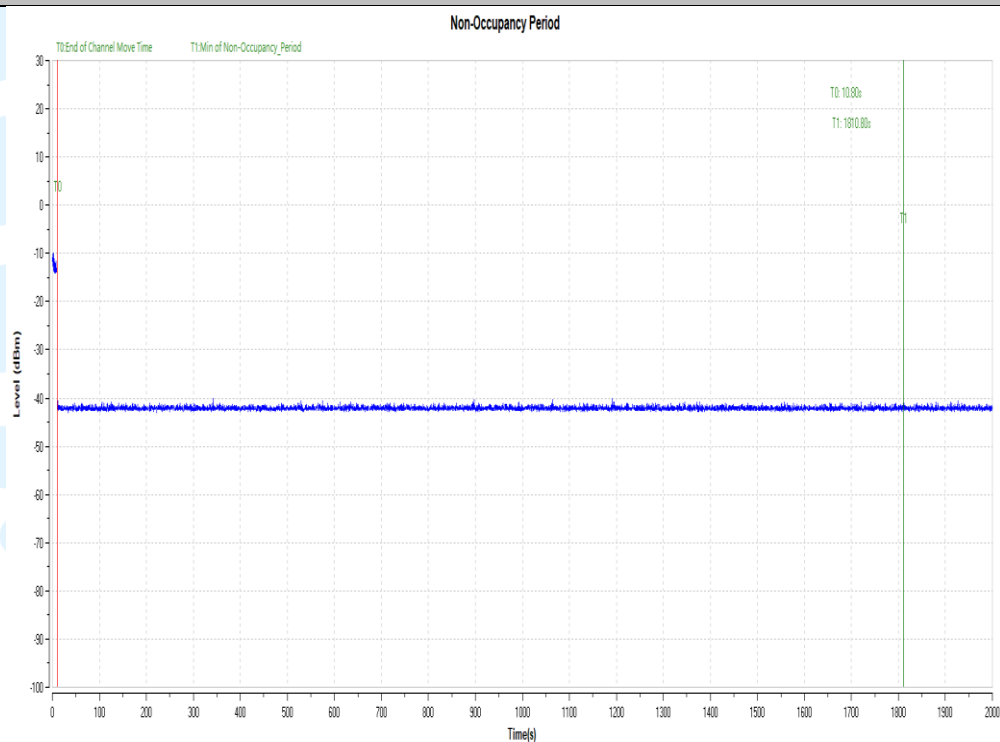
11AC80SISO-5530-Type0-PASS
