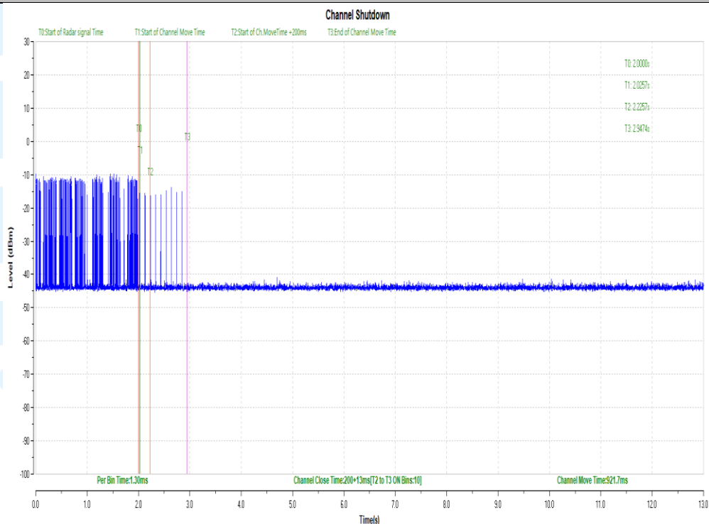
11AC80SISO-5530-Type0-PASS
