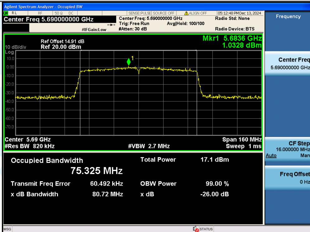
11AC80SISO-Ant1-5690
