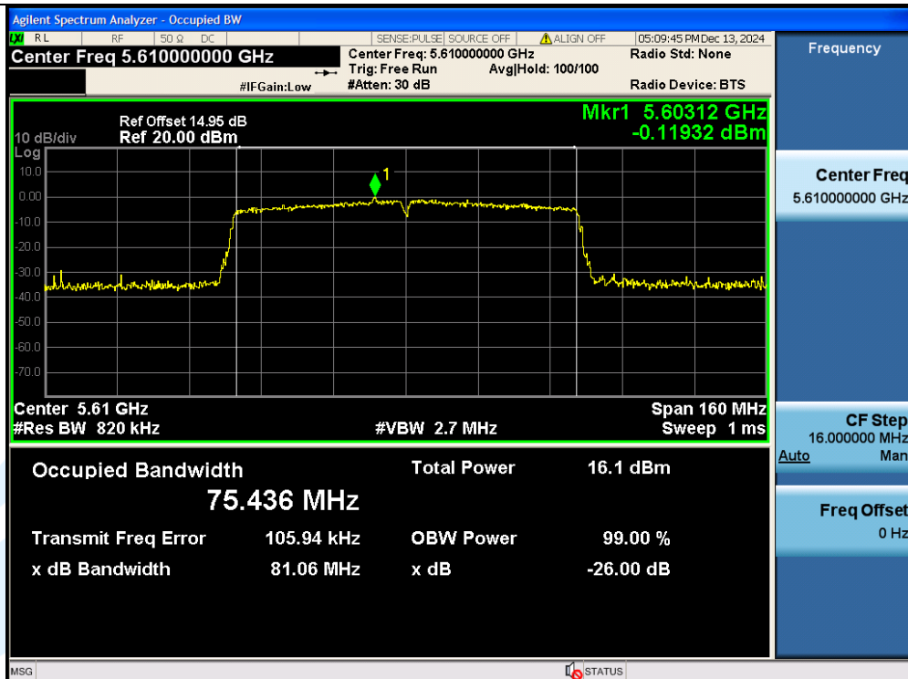
11AC80SISO-Ant1-5610
