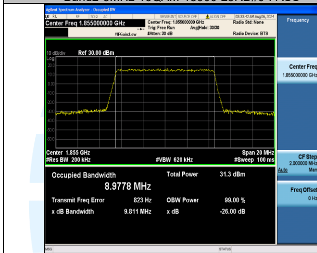
Band2-10MHz-QPSK-18650-50RB#0-PASS
