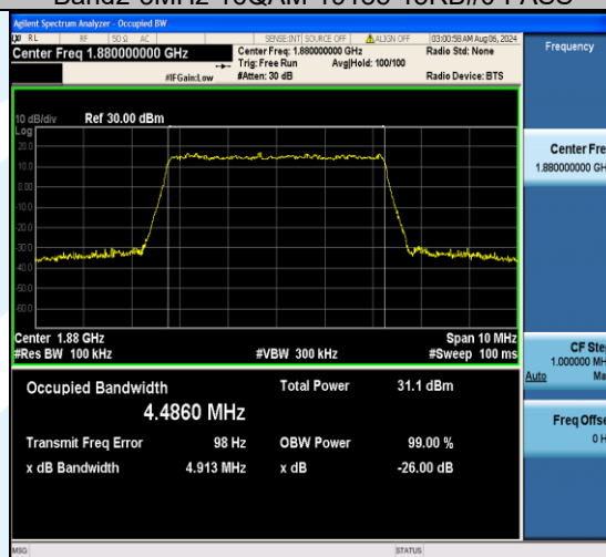
Band2-5MHz-QPSK-18900-25RB#0-PASS
