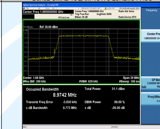
Band2-10MHz-QPSK-18900-50RB#0-PASS
