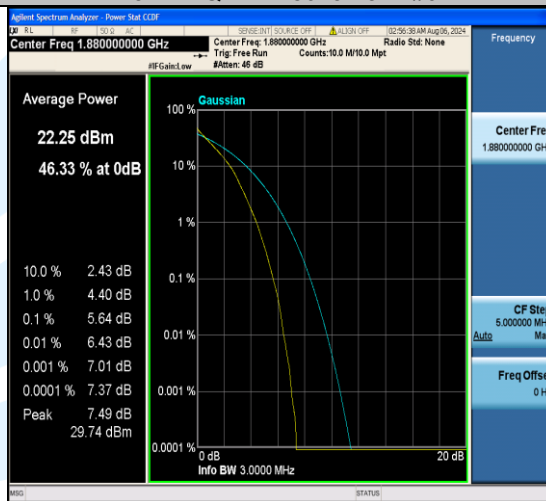
Band2-3MHz-QPSK-18900-15RB#0-PASS
