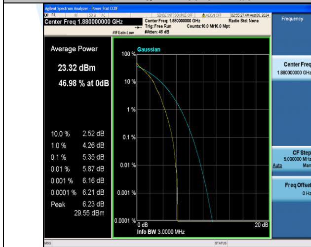
Band2-3MHz-QPSK-18900-1RB#0-PASS
