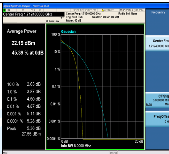
Band4-1312-1-PASS
