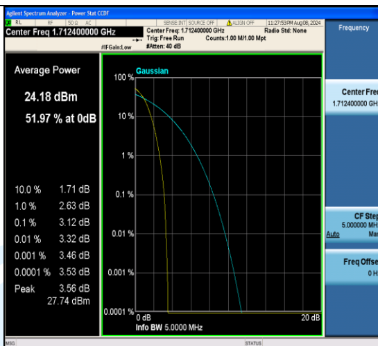
Band4-1312-1-PASS
