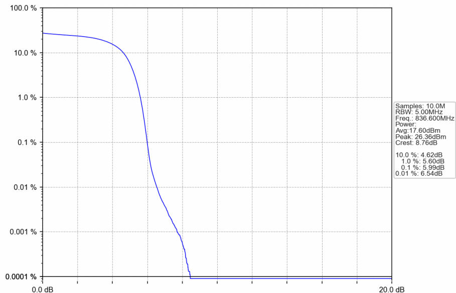
Band5_HSUPA_MCH_836.6MHz_Subtest 1_NTNV
