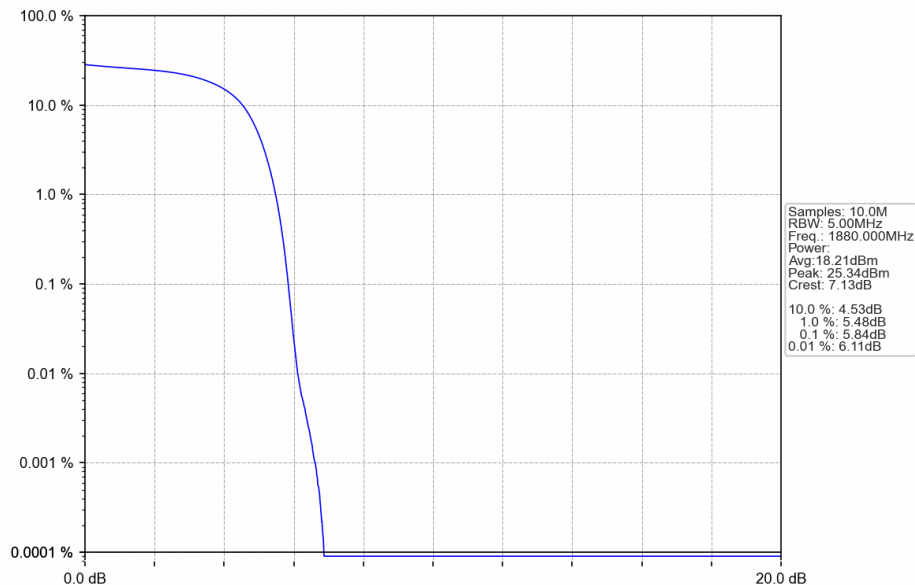
Band2_HSUPA_MCH_1880MHz_Subtest 1_NTNV
