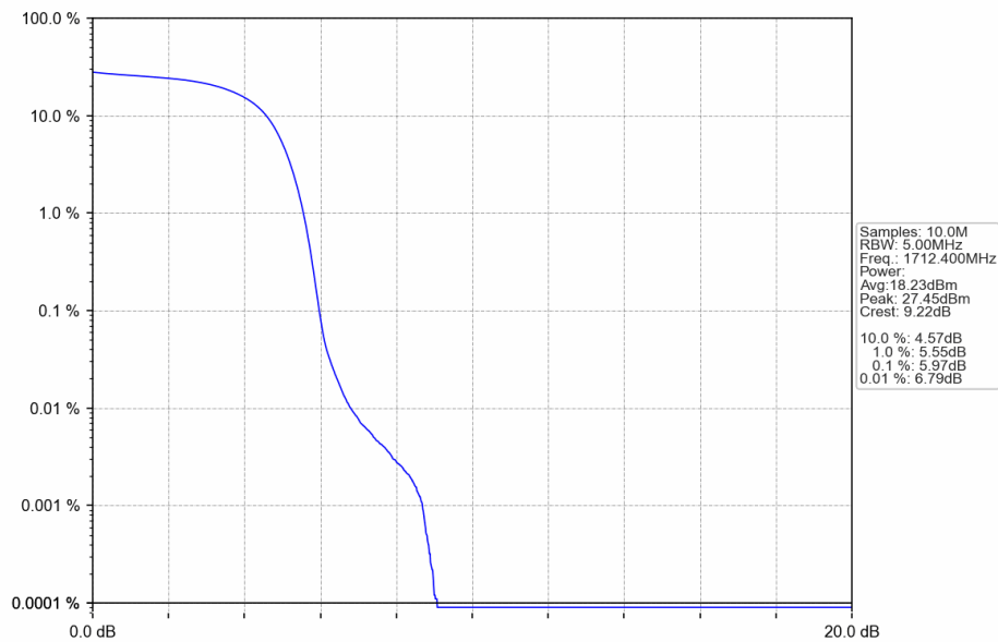
Band4_HSUPA_LCH_1712.4MHz_Subtest 1_NTNV
