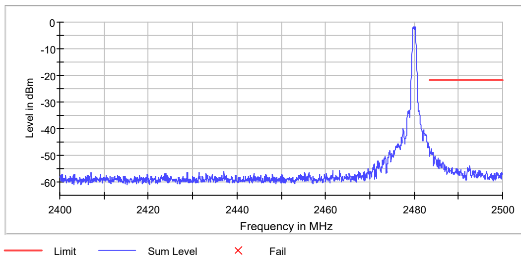
Band Edge
