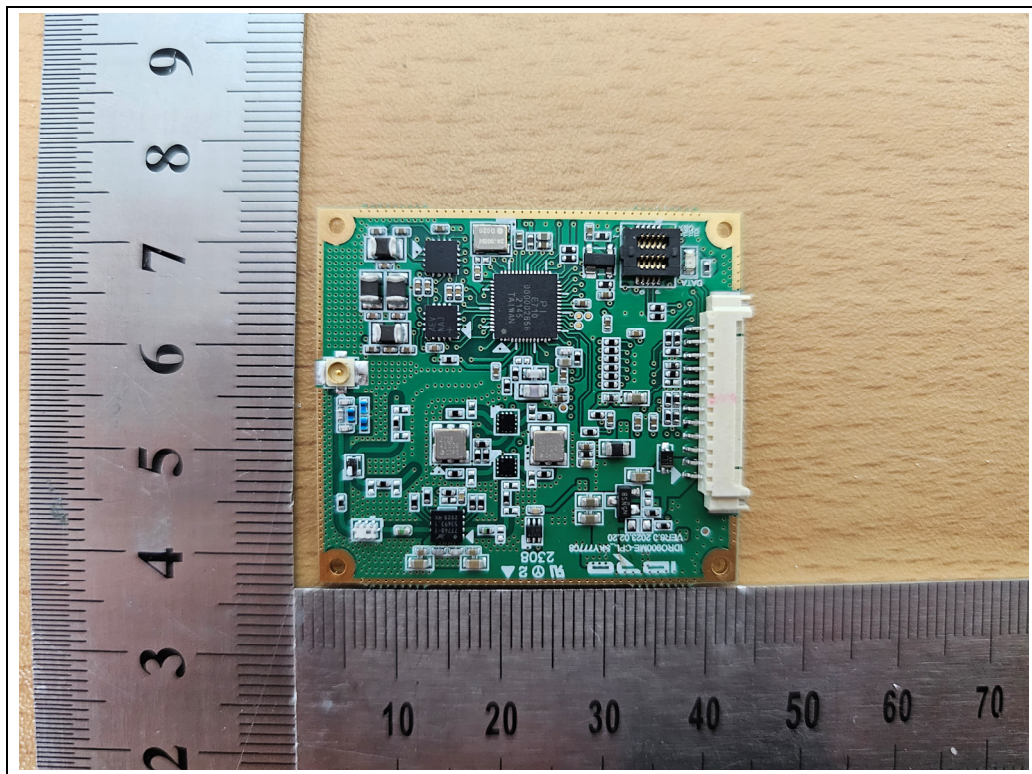
<RFID Module>
