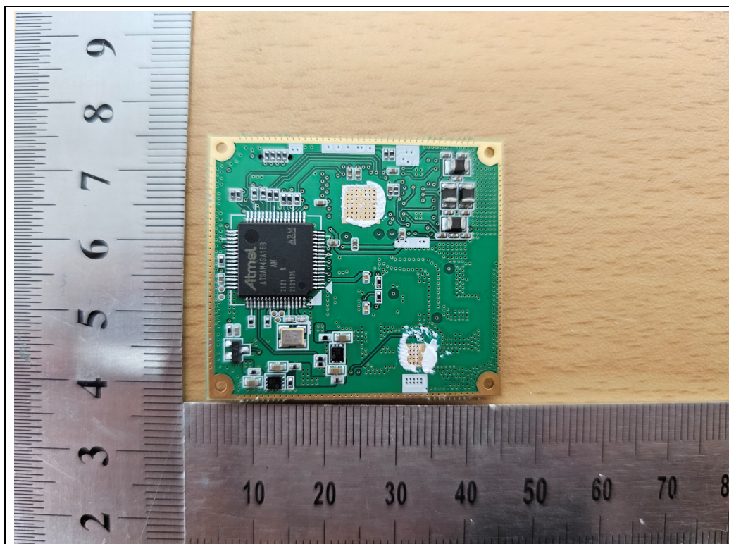
<RFID Module>
