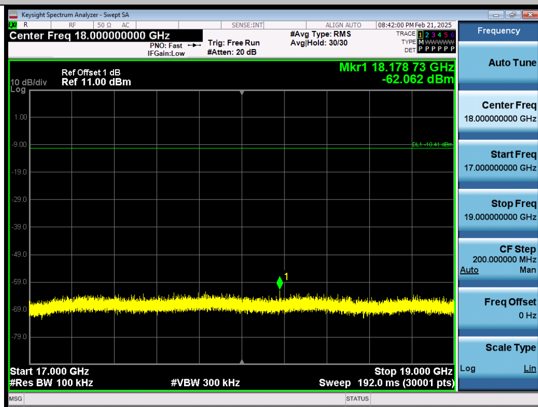
DH5-Ant1-2441-17000~19000-PASS
