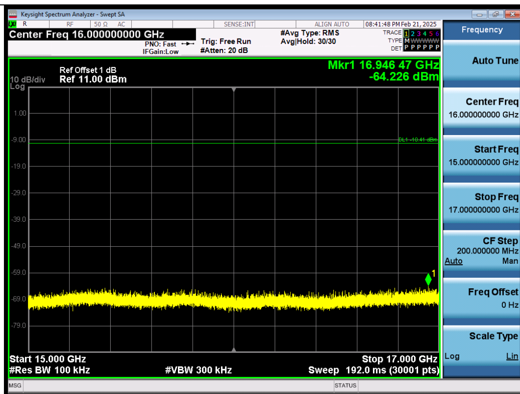
DH5-Ant1-2441-15000~17000-PASS
