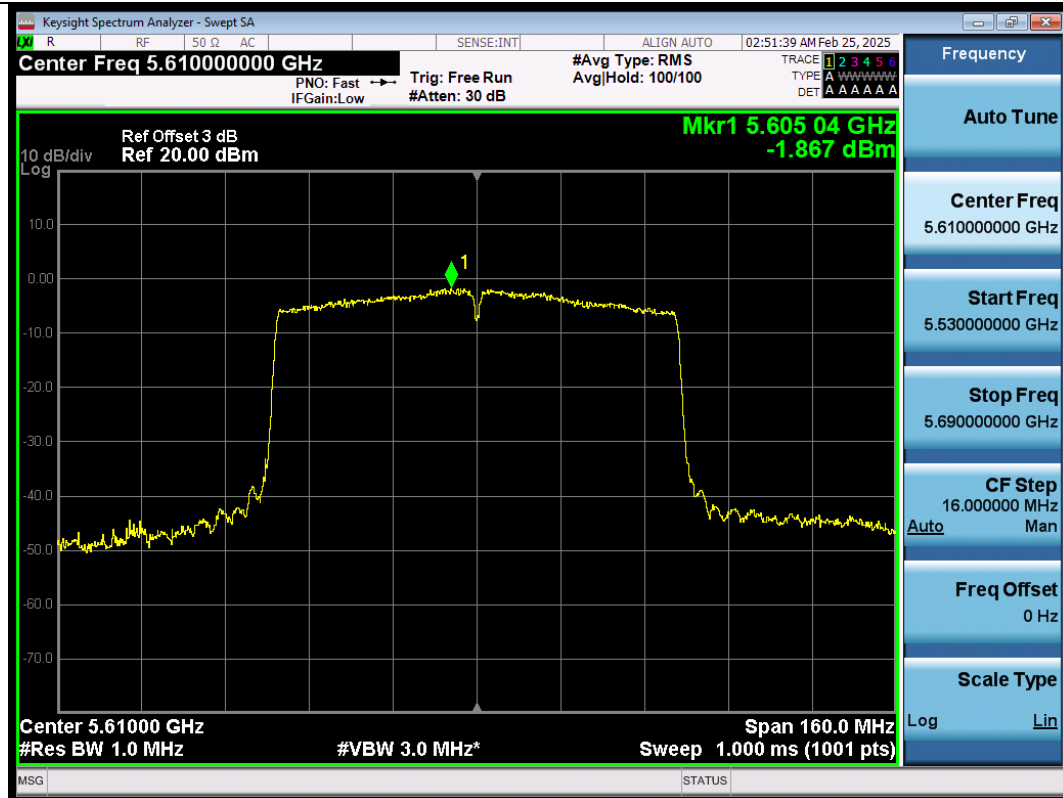
11AC80SISO-Ant1-5610-PASS
