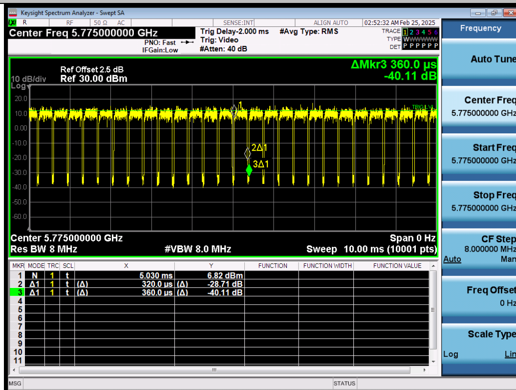
NTNV-11AC80SISO-Ant1-5775
