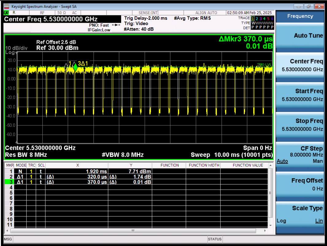
NTNV-11AC80SISO-Ant1-5530
