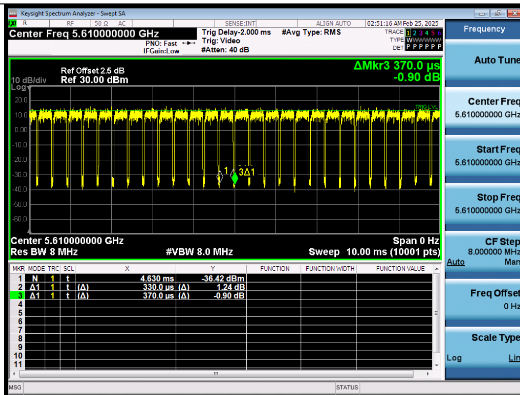
NTNV-11AC80SISO-Ant1-5610
