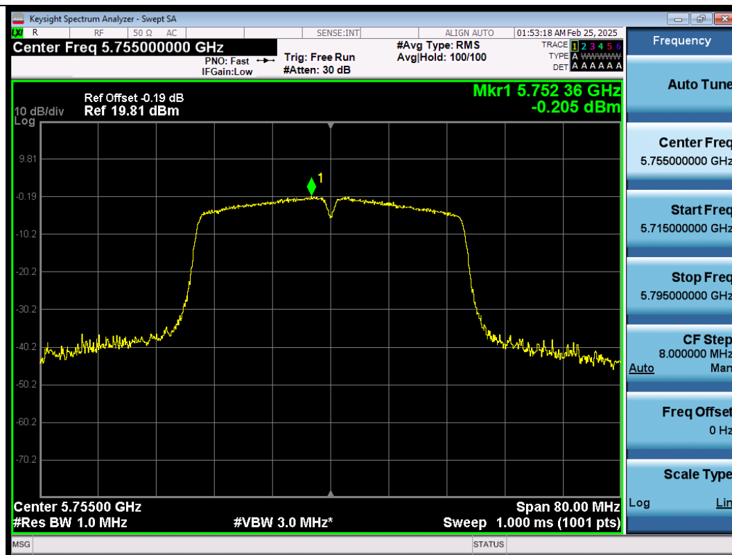
11N40SISO-Ant1-5755-PASS
