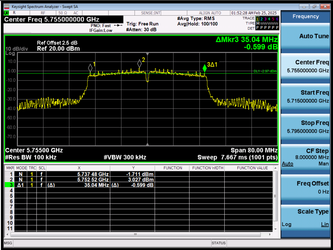
11N40SISO-Ant1-5755-PASS
