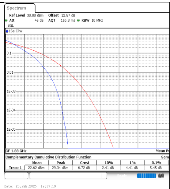
Band2-10MHz-QPSK-18900-50RB#0-PASS
