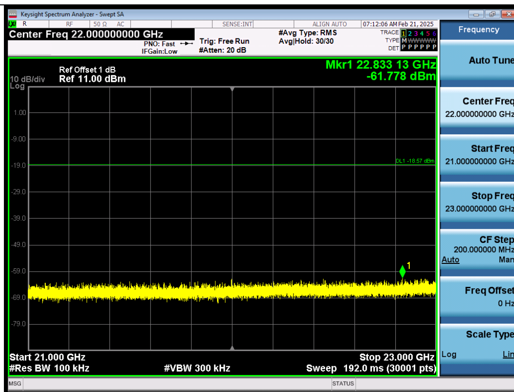
BLE_2M-Ant1-2404-21000~23000-PASS
