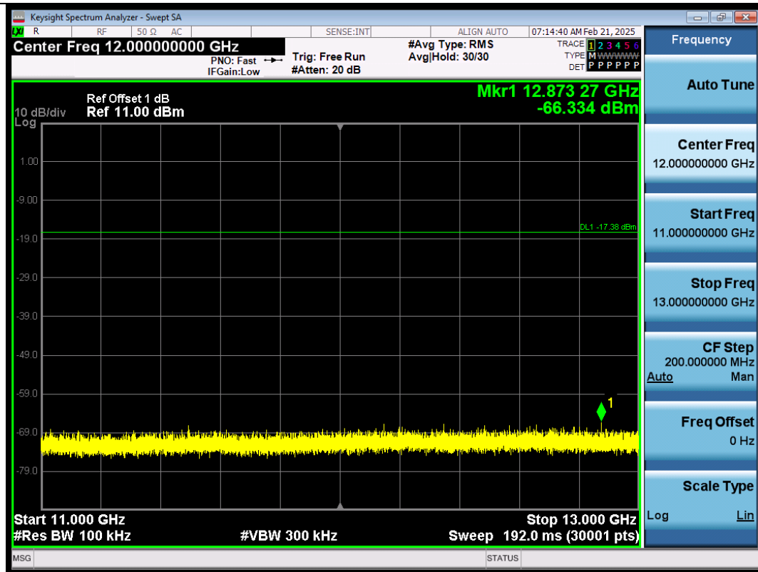
BLE_2M-Ant1-2440-11000~13000-PASS
