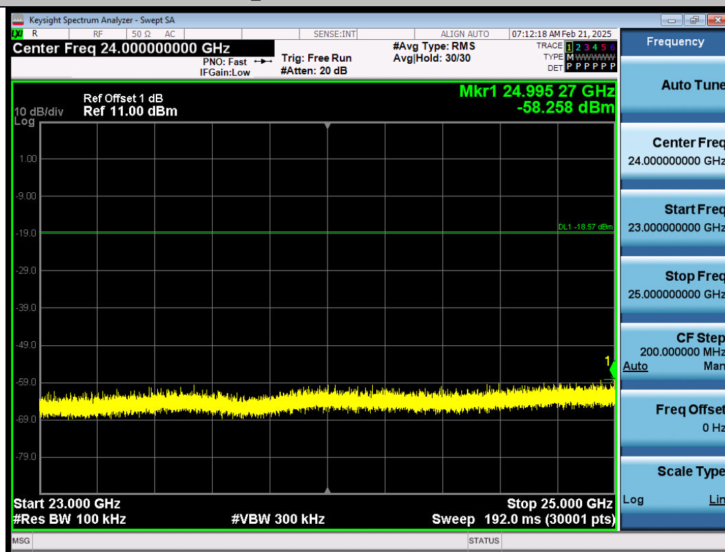
BLE_2M-Ant1-2404-23000~25000-PASS
