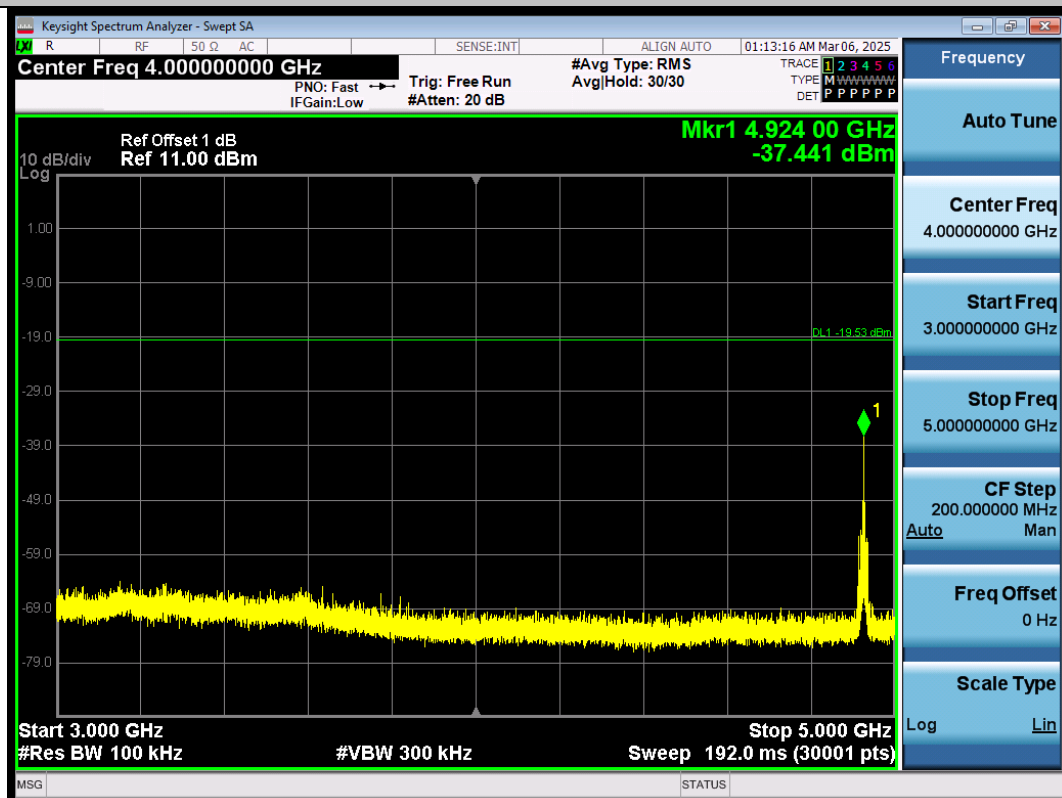
11B-Ant1-2462-3000~5000-PASS
