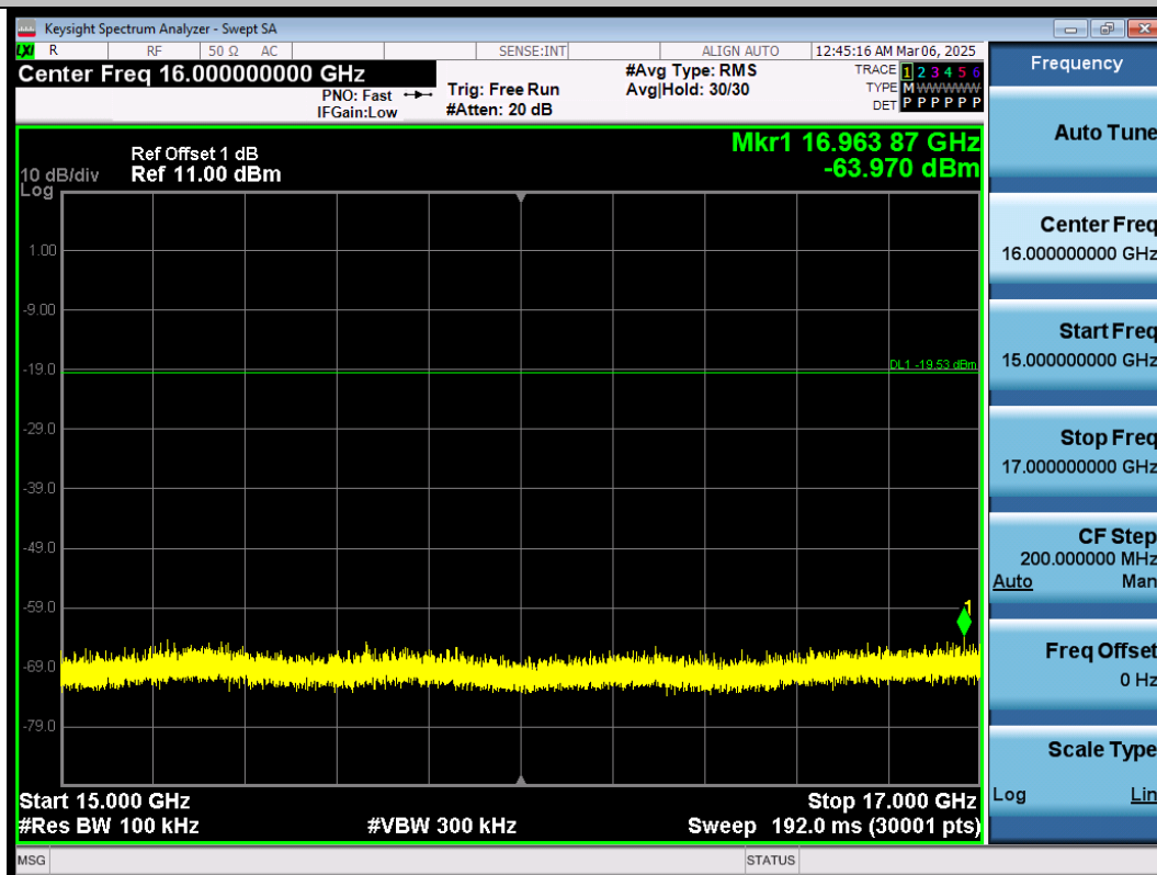
11B-Ant1-2412-15000~17000-PASS
