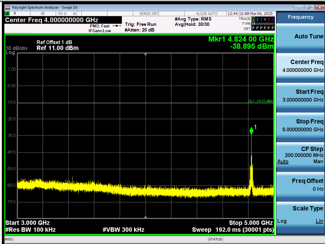
11B-Ant1-2412-3000~5000-PASS
