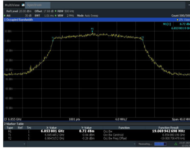
11AX20SISO_Ant2_6855
