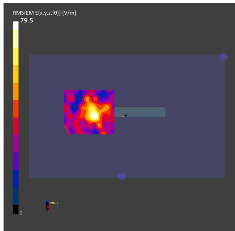
Fig. 3 WLAN 6GHz PD
