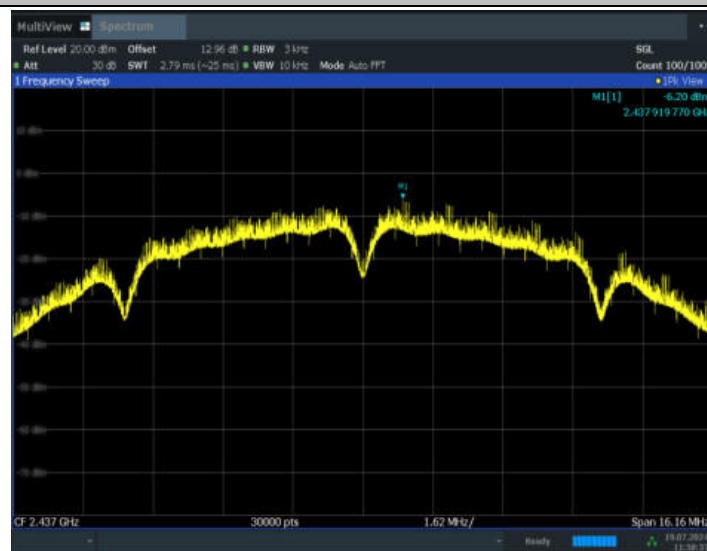
11B_Ant2_2437
