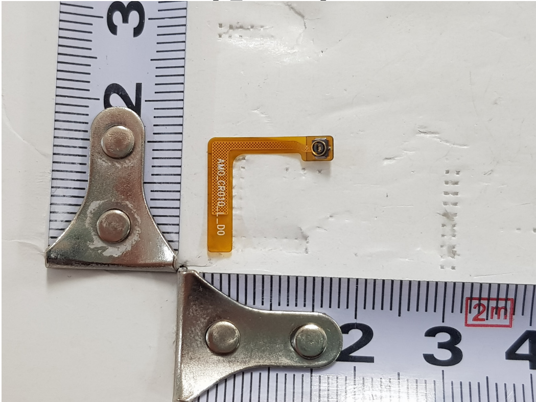
[L_Antenna]
