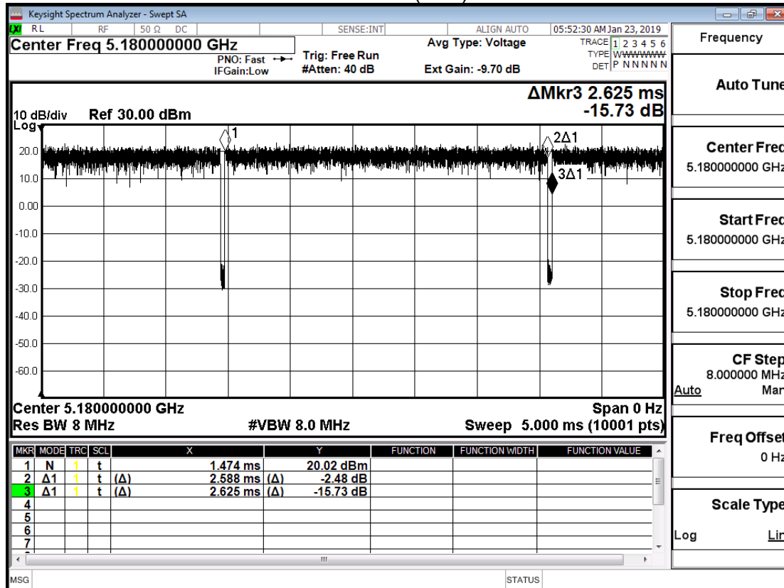
802.11ac(20M)
