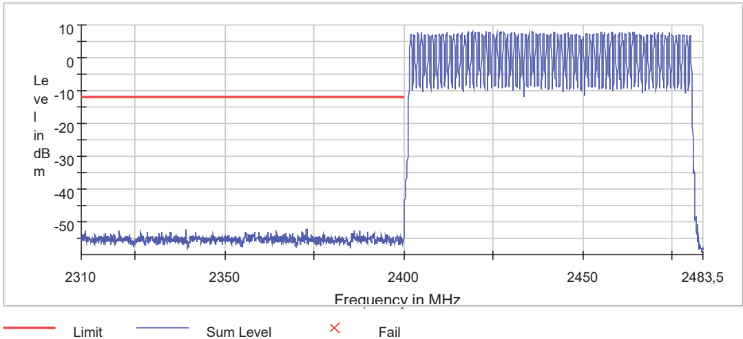
Band Edge
