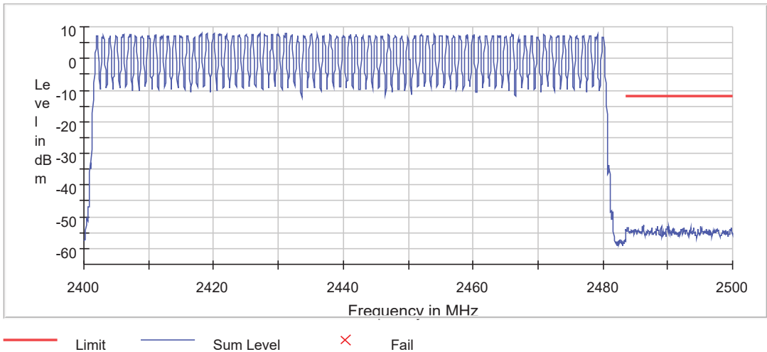
Band Edge
