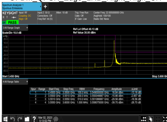
N77(20M)_CP- OFDM_QPSK Edge 1RB Right High CH
