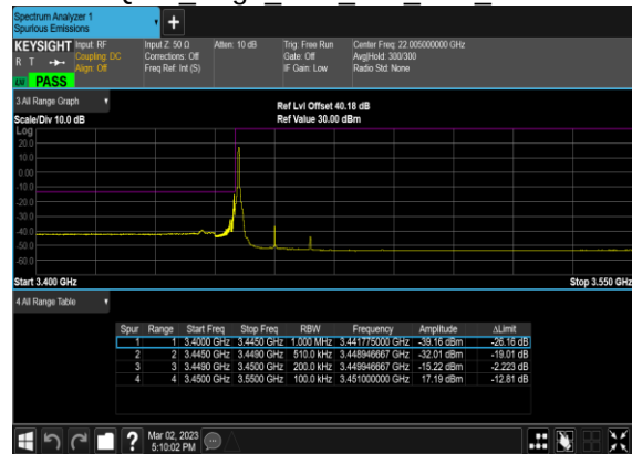
N77(20M)_CP-OFDM_16 QAM Edge 1RB Left Low CH
