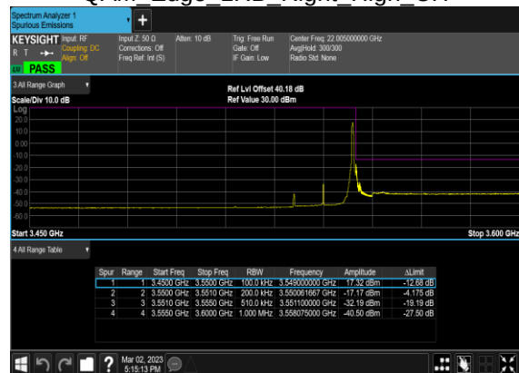
N77(20M)_CP-OFDM_16 QAM Edge 1RB Right High CH
