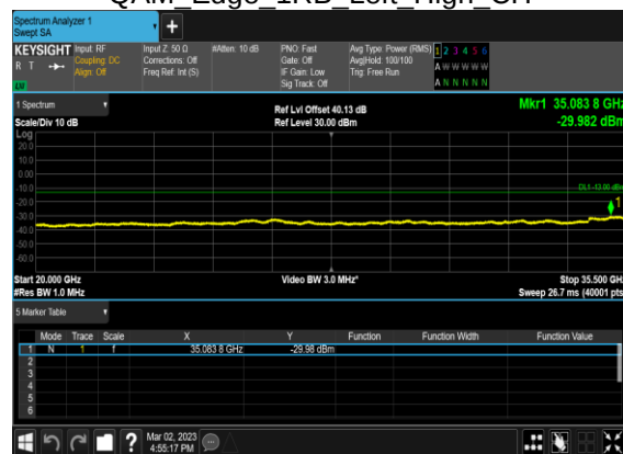
N77(20M)_CP-OFDM_16 QAM Edge 1RB Left High CH
