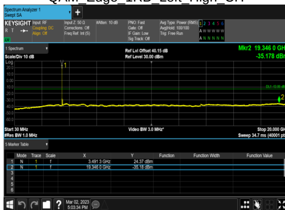
N77(60M)_CP-OFDM_16 QAM Edge 1RB Left High CH
