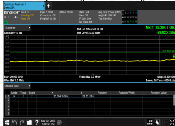
N77(60M)_CP- OFDM QPSK Edge 1RB Left High CH
