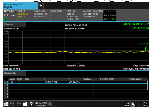
N77(60M)_CP- OFDM QPSK Edge 1RB Left Mid CH
