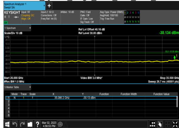
N77(60M)_CP- OFDM QPSK Edge 1RB Left Low CH
