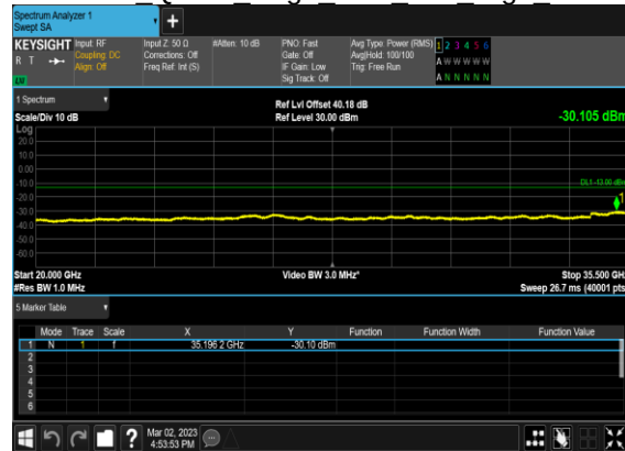
N77(20M)_CP- OFDM QPSK Edge 1RB Left High CH
