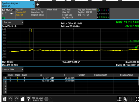
N77(60M)_CP- OFDM QPSK Edge 1RB Left Low CH
