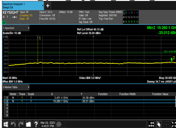
N77(20M)_CP- OFDM QPSK Edge 1RB Left Low CH
