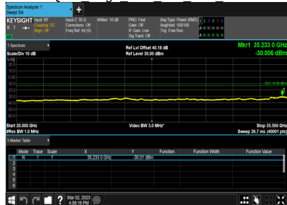
N77(60M)_CP-OFDM_16 QAM Edge 1RB Left Low CH
