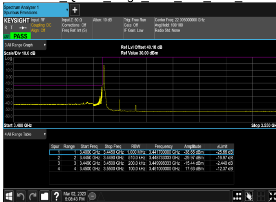
N77(20M)_CP- OFDM_QPSK Edge 1RB Left Low CH
