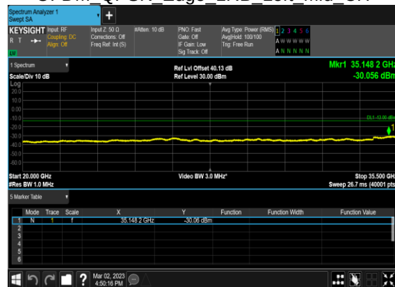
N77(20M)_CP- OFDM QPSK Edge 1RB Left Mid CH
