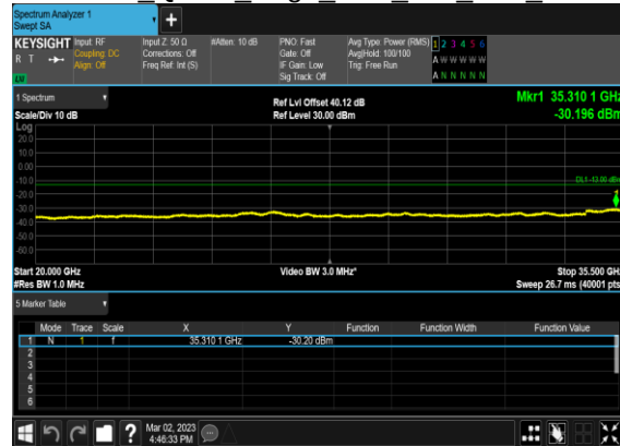
N77(20M)_CP- OFDM QPSK Edge 1RB Left Low CH
