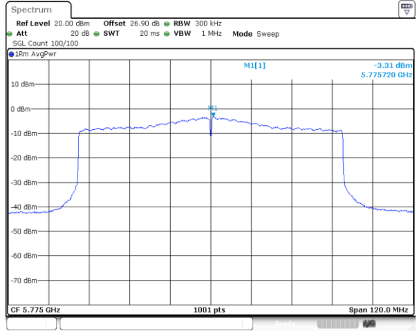
MIMO Ant. 7
