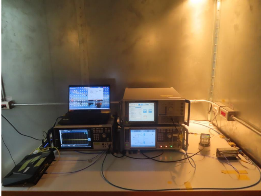
EUT
