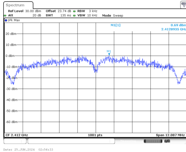
MIMO Ant 1
