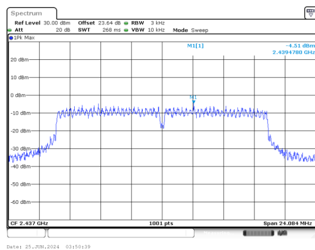
MIMO Ant 1
