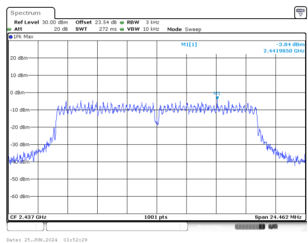
MIMO Ant 2
