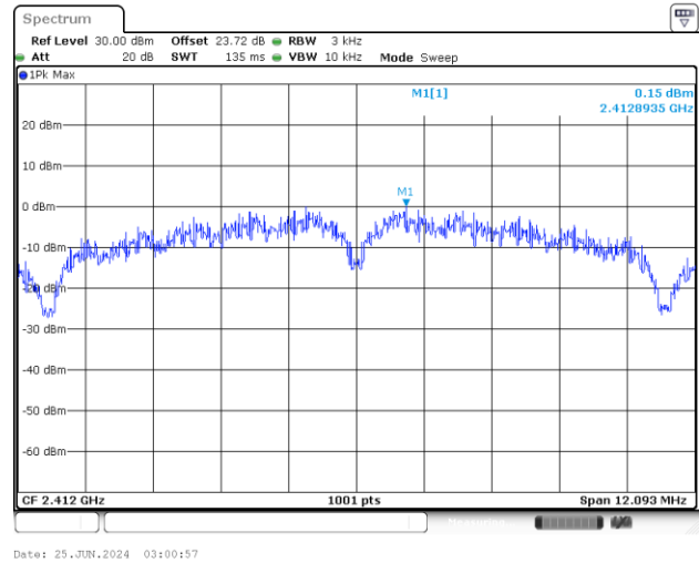
MIMO Ant 2
