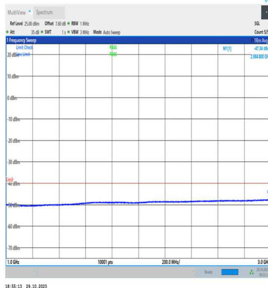
NTVN_N48_PC3_30_30_L_TID1_NS_01_1000_3000_#1
