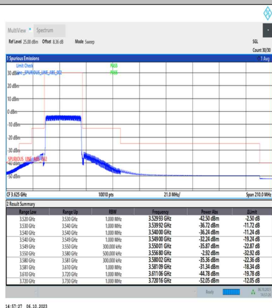
NTNV_N48_PC3_30_30_L_TID6_RID1#1
