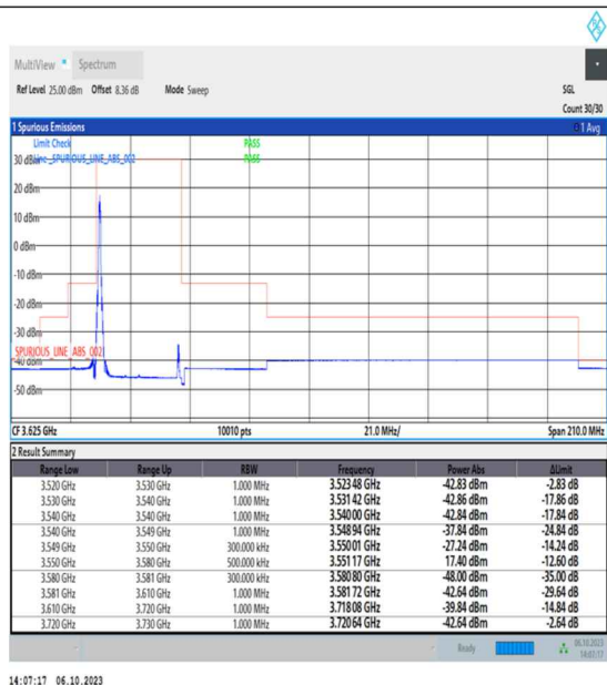
NTNV_N48_PC3_30_30_L_TID1_RID1#1
