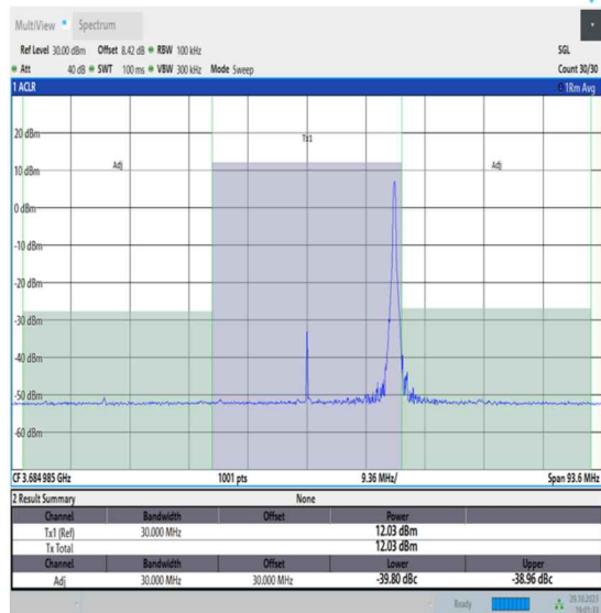
NTNV_N48_PC3_30_30_H_TID18_#1_-30_30
