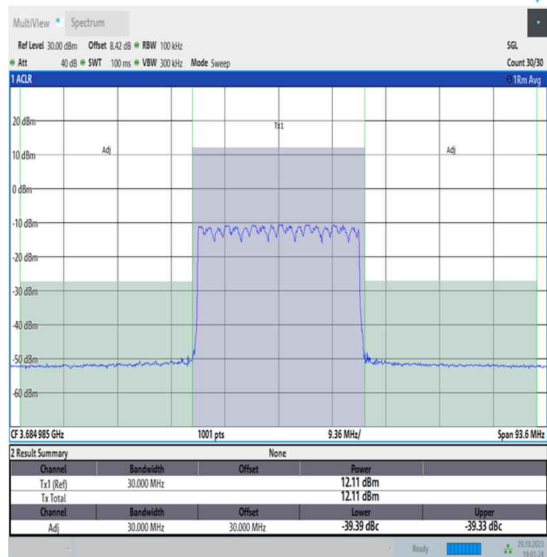
NTNV_N48_PC3_30_30_H_TID16_#1_-30_30
