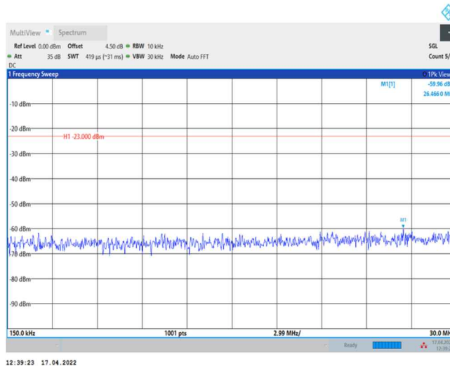
Band12-10MHz-QPSK-23060-1RB#0-Range2:0.15~30MHz
