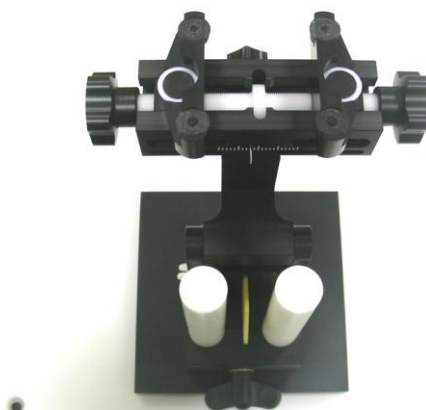
Fig. 5.10 Phone Positioner
