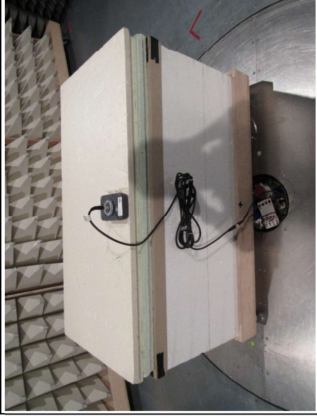
EUT Test Setup
