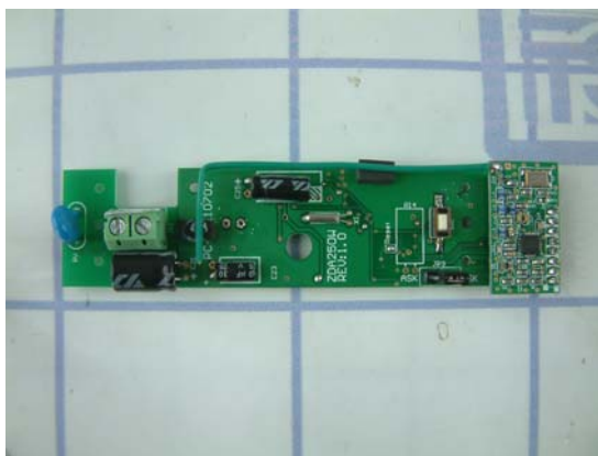
ZDA250W PCB side 2
