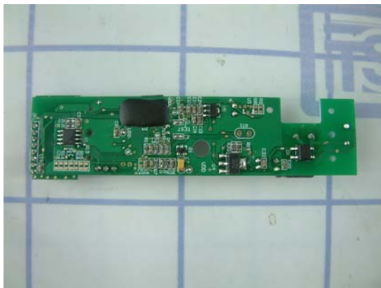
ZDA250W PCB side 1
