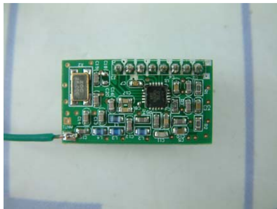
Z270W Module side 1
